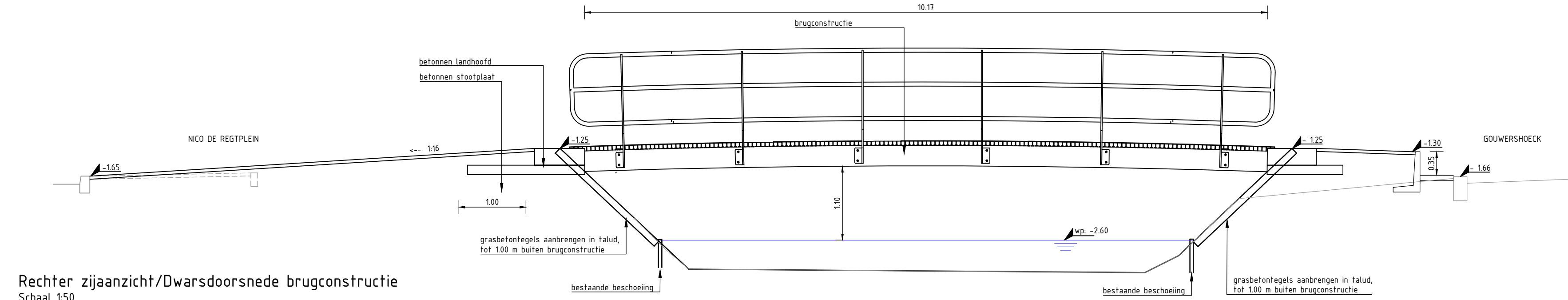
Situatie overzicht Schaal 1:100
