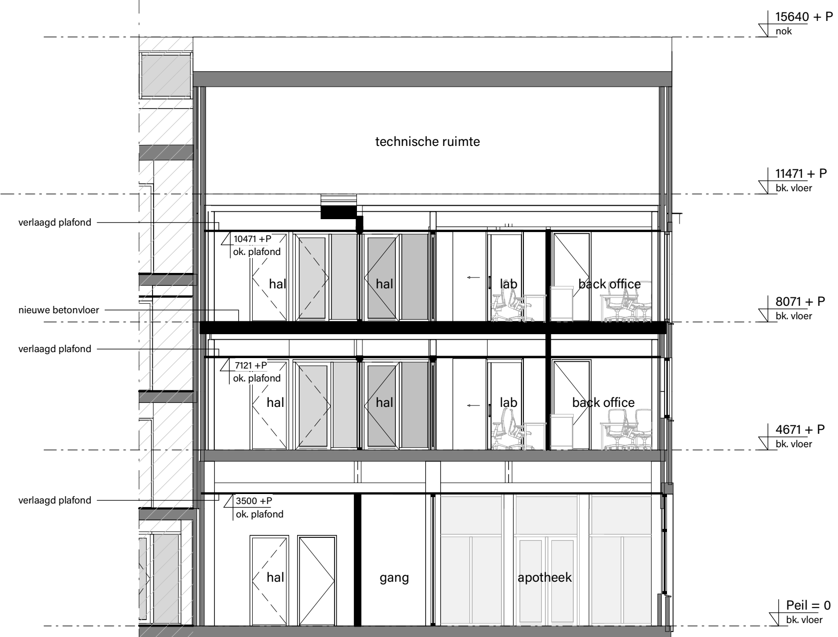
Doorsnede A-A
