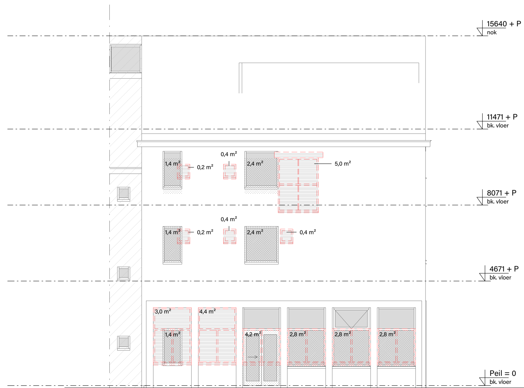
Voorgevel
