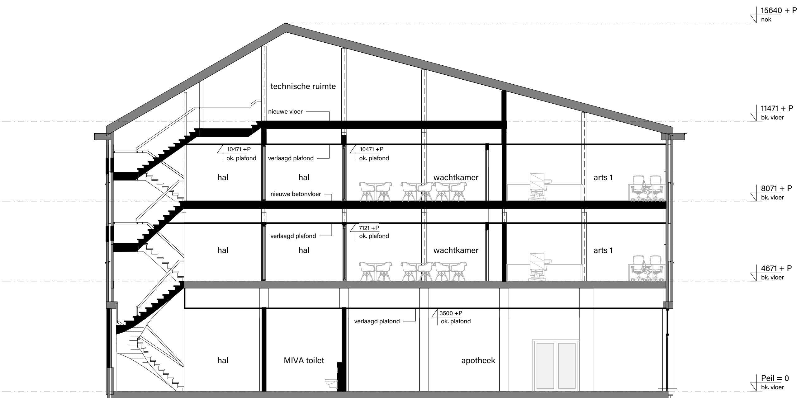
Doorsnede B-B
