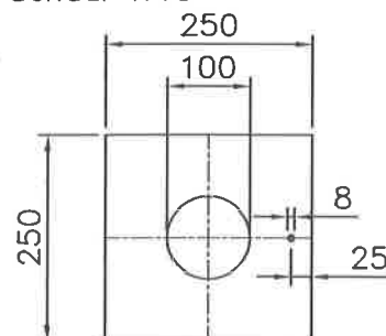
DETAIL GRONDPLAAT Schaal 1:10
