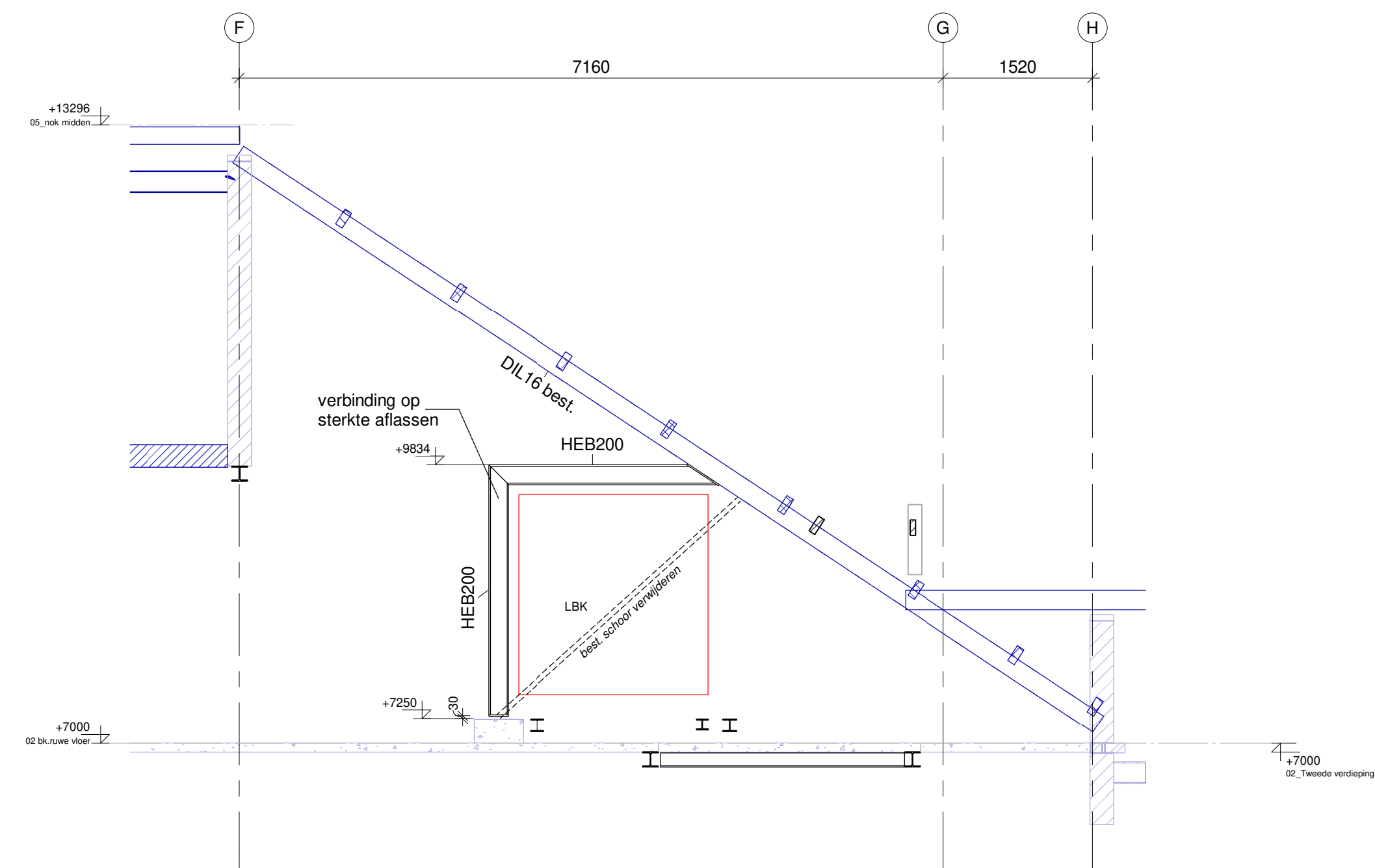
Aanzicht 1/2 stalen spant best.
