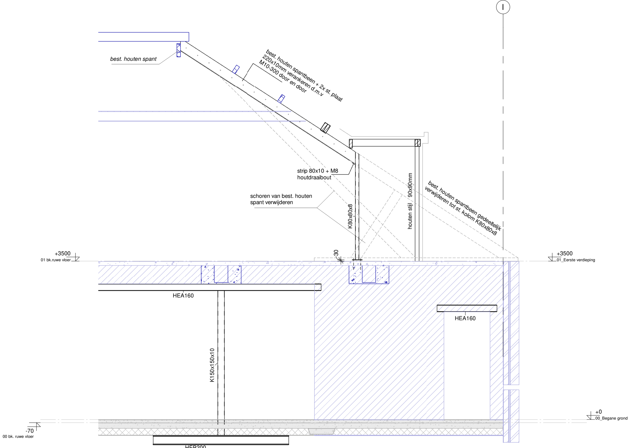
Aanzicht houten 1/2 spant 2 best
