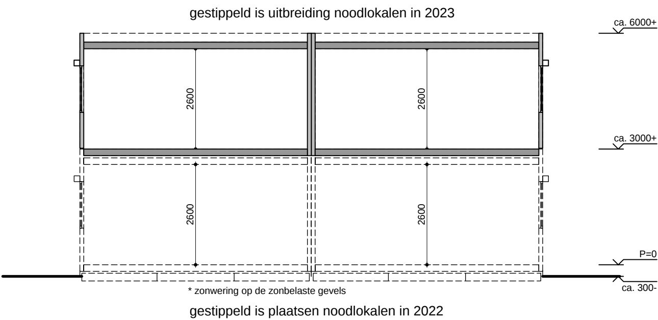
Dwarsdoorsnede
