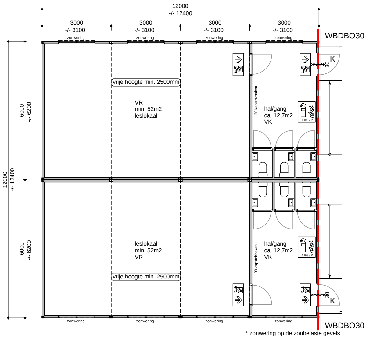
1e verdieping
