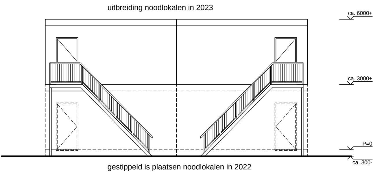
Rechter-zijgevel (WBDBO30)
