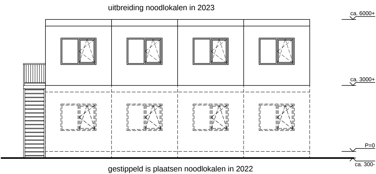
Achtergevel
