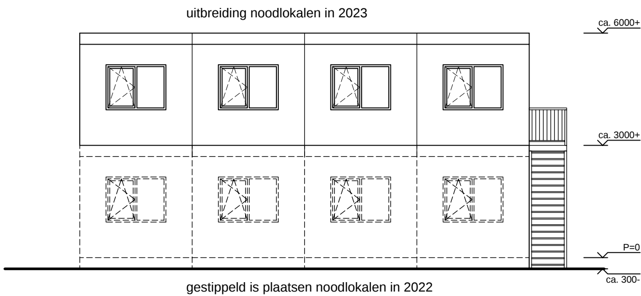
Voorgevel
