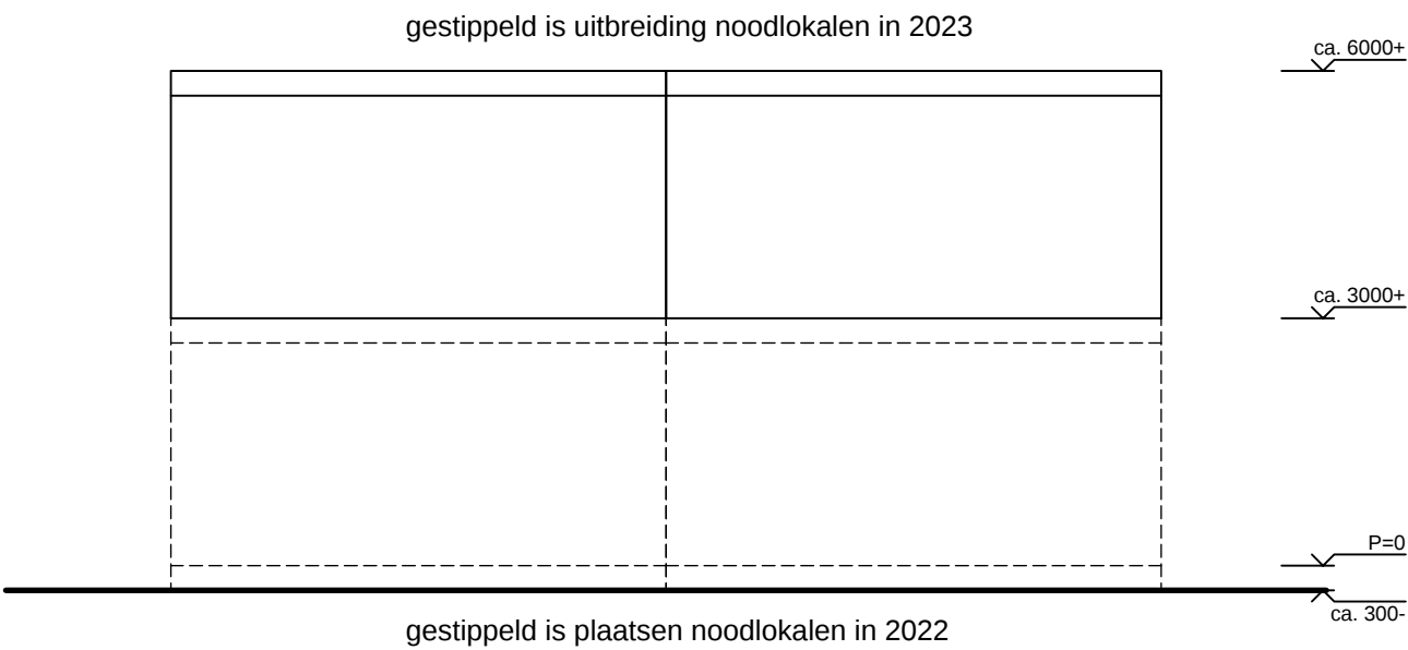
Linker-zijgevel
