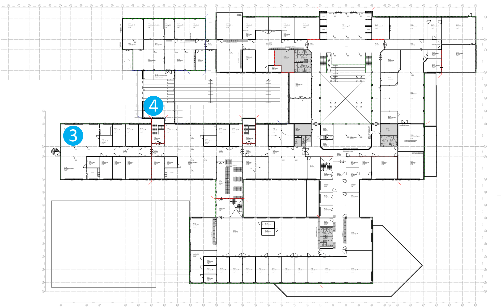
VERDIEPING NIEUW (2022)
