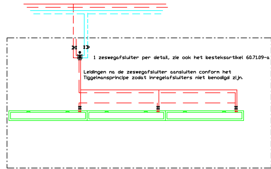
DETAIL 1: Het aansluitprincipe inductieunits o.b.v. een zeswegafsluiter.
