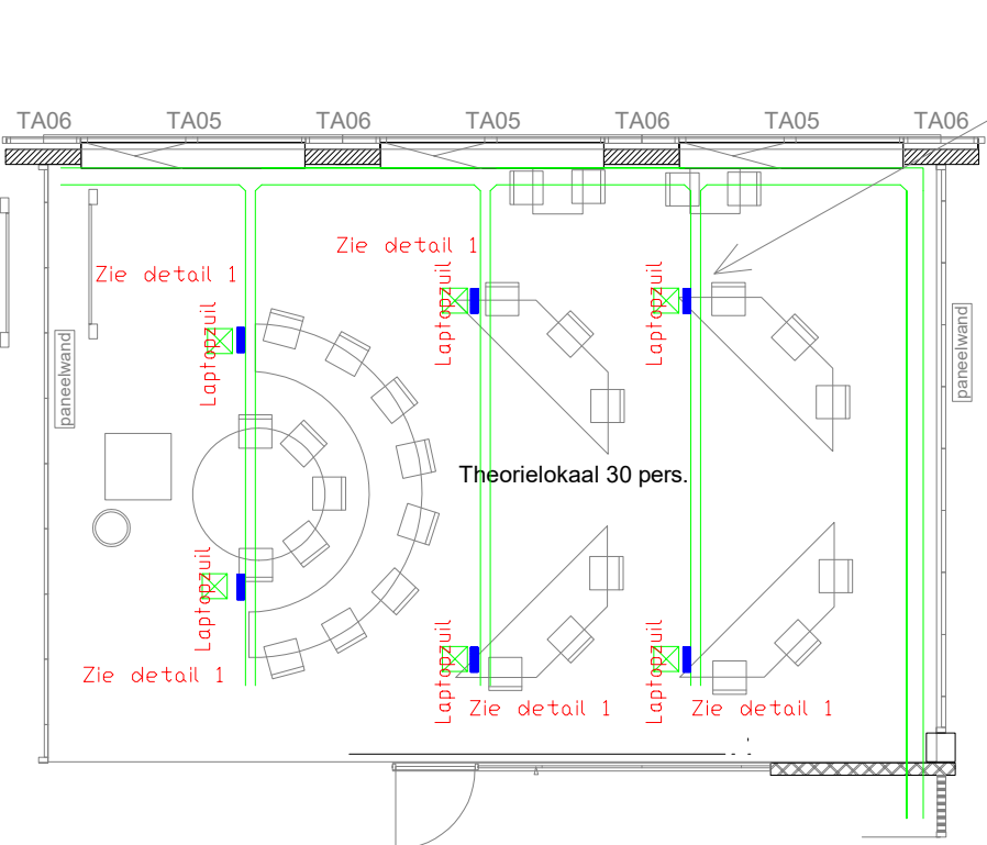
Detail 1 komt bij elke laptopzuil terug welke een dataoutlets bezitten
