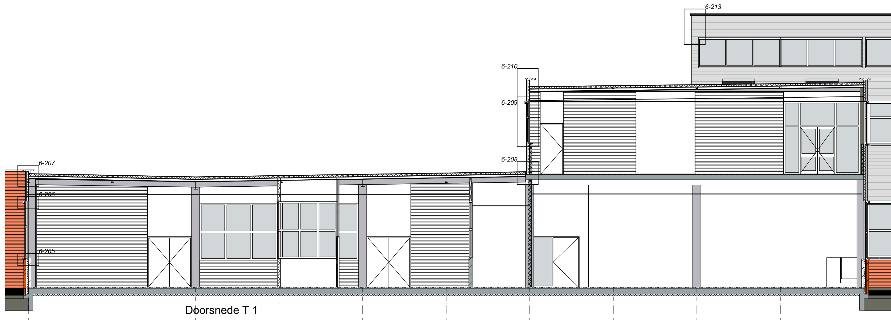
Doorsnede T 1
