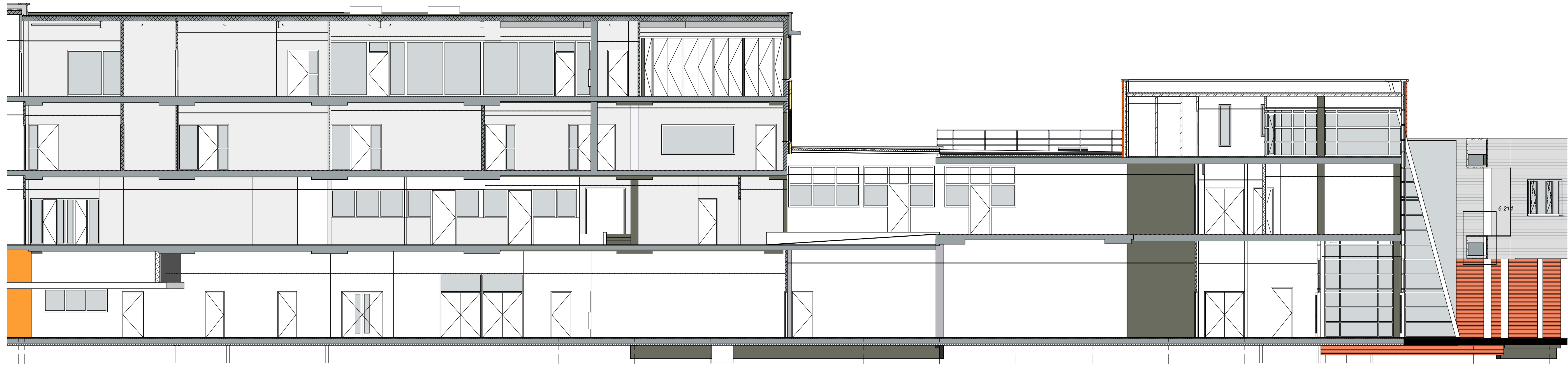
Doorsnede T 3
