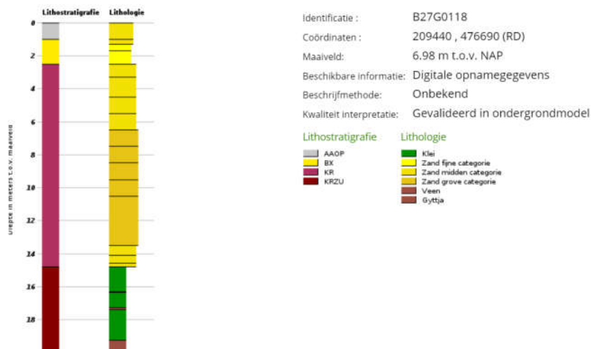
Afbeelding 2.1: Boorbeschrijving boring B27G00118
