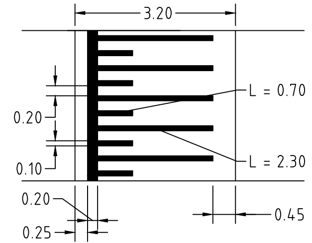
Plateau 60 km/u, hoogte 80 mm
