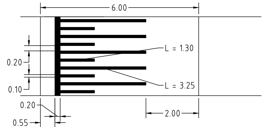
Plateau 60 km/u, hoogte 120 mm
