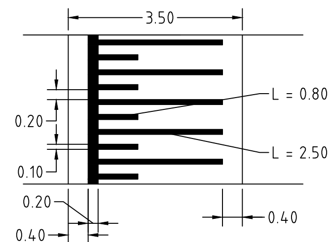
Plateau 50 km/u, hoogte 120 mm
