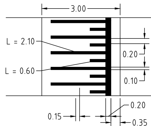
Drempel 50 km/u, hoogte 80 mm
