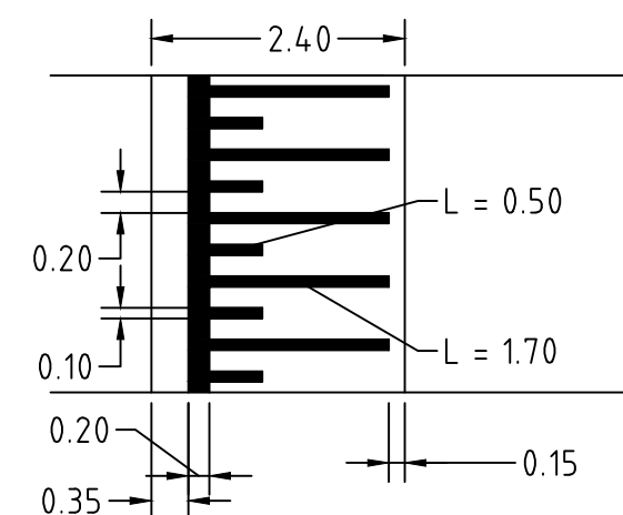
Plateau 50 km/u, hoogte 80 mm
