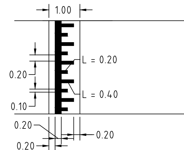
Plateau 30 km/u, hoogte 80 mm
