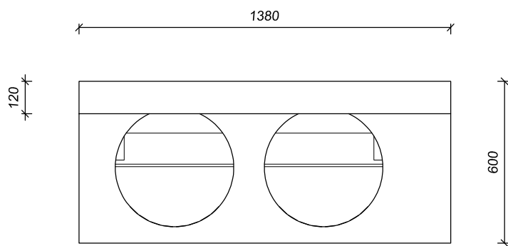
Bovenaanzicht
