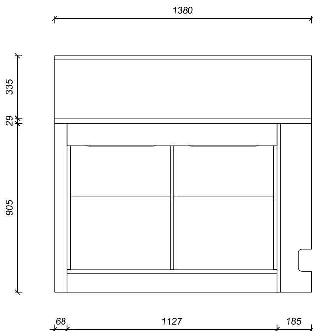
Vooraanzicht
