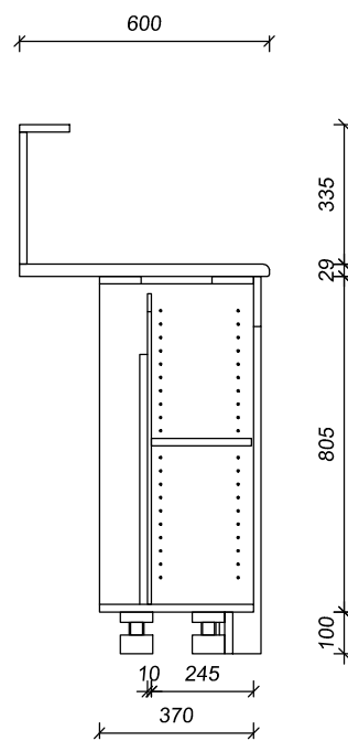
Doorsnede
