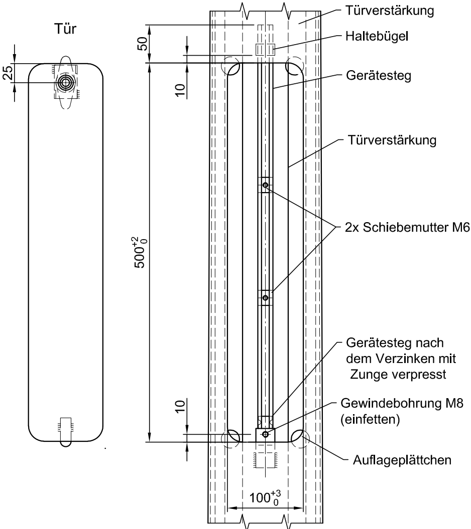
Detail Türausschnitt M1:5
