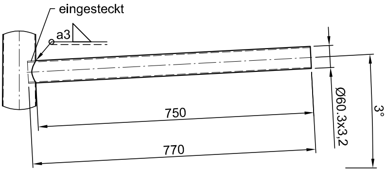
Detail Stutzen M1:10
