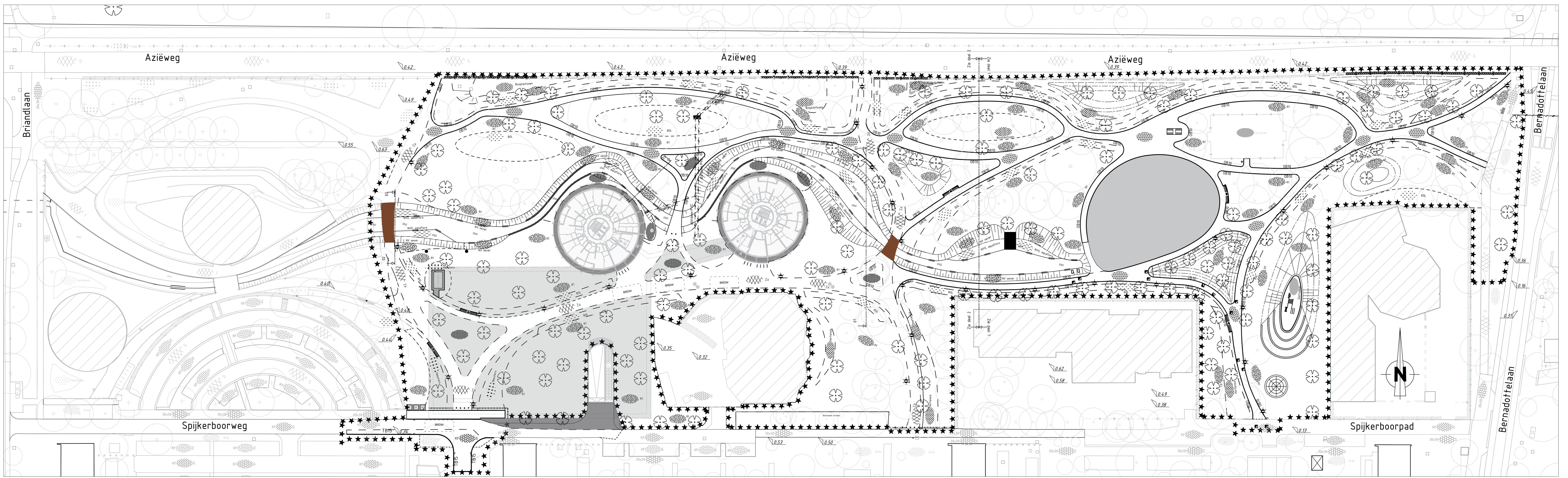
NIEUWE SITUATIE SCHAAL 1:500
