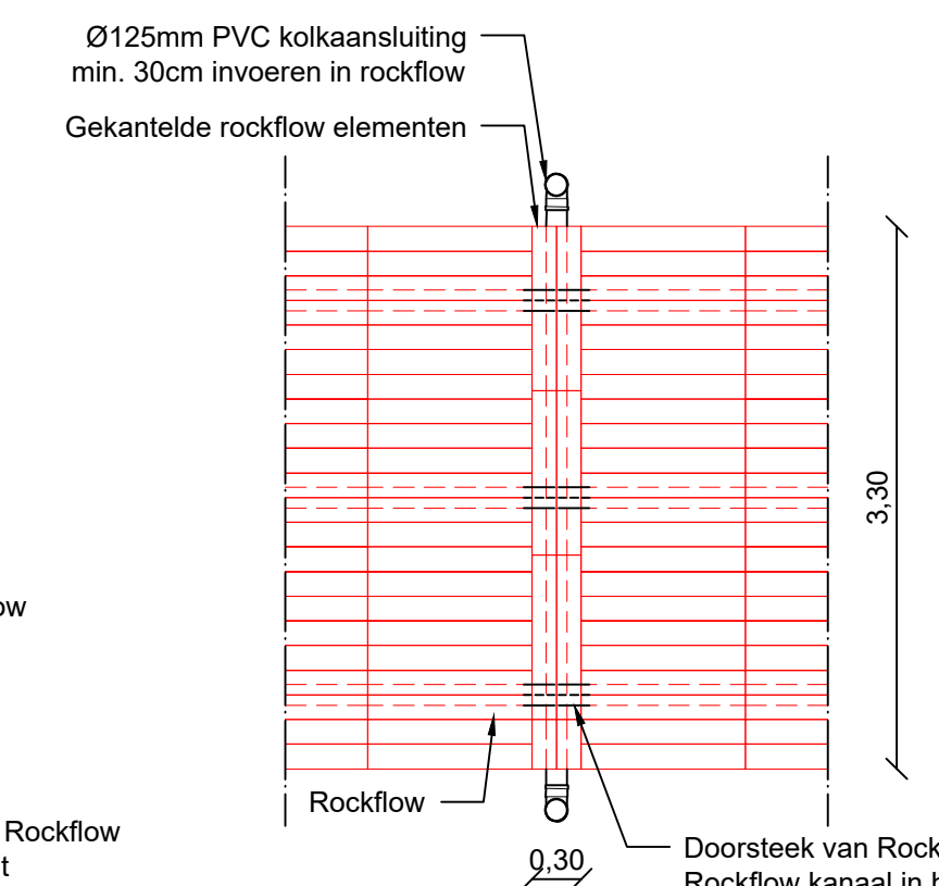
Detail Q: Aansluiting kolken op Rockflow Bovenaanzicht Schaal: 1:50
