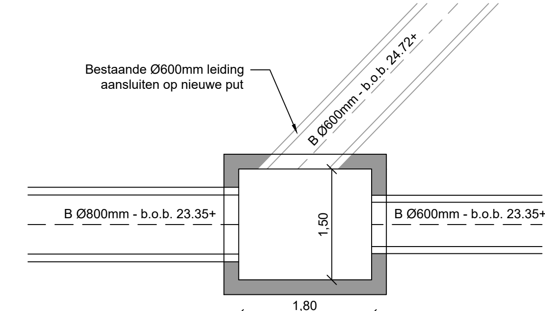
Detail K: Put 05572 Bovenaanzicht Schaal: 1:50
