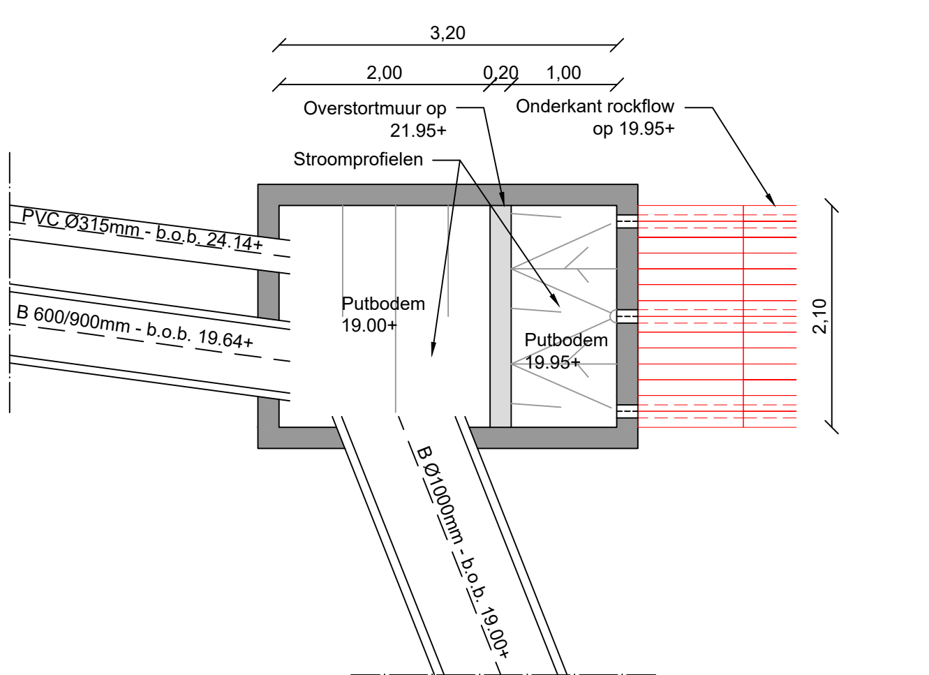
Detail S: Put 05508 Bovenaanzicht Schaal: 1:50
