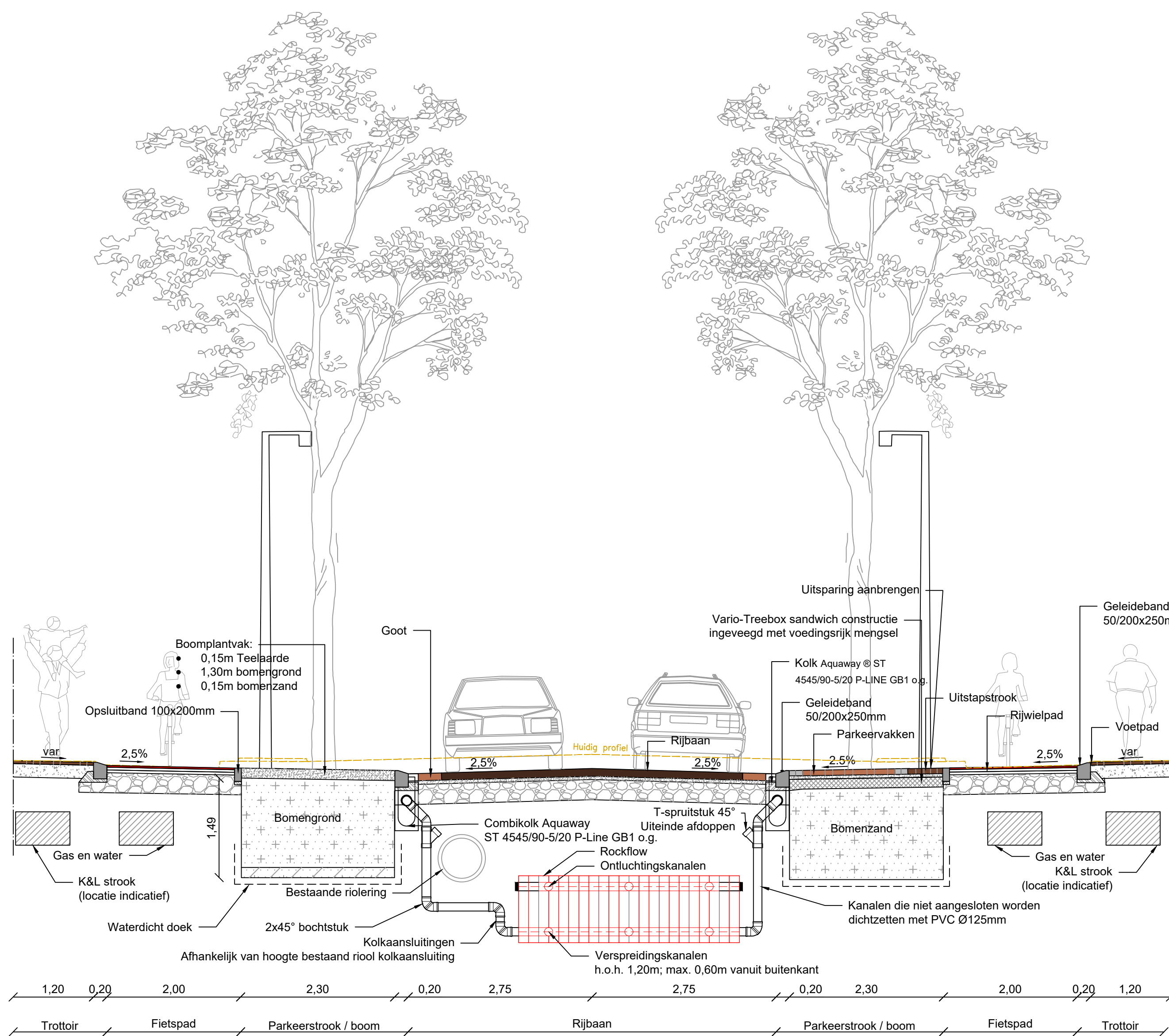
Principeprofiel: Kapellerlaan Zijaanzicht Schaal: 1:50
