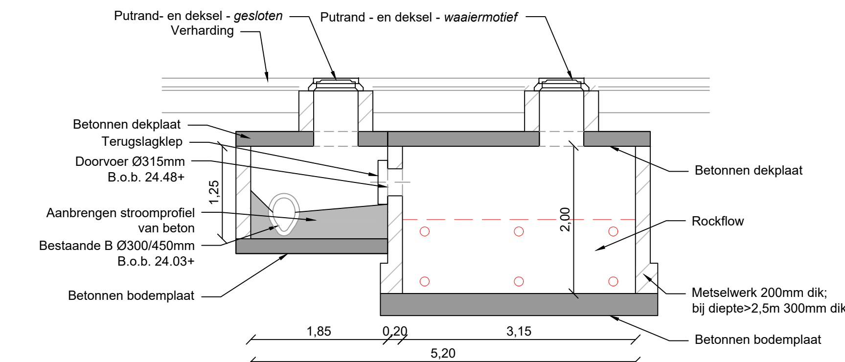
Detail J: Put 05502 Zijaanzicht Schaal: 1:50
