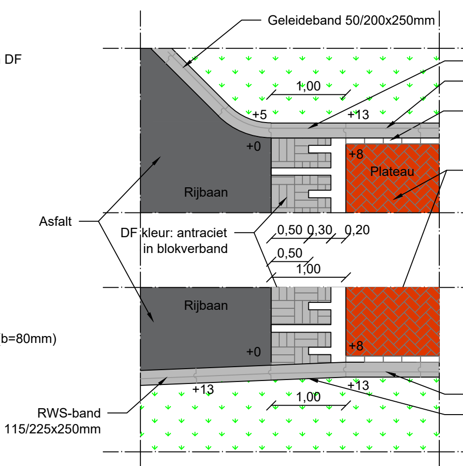
Detail F: Oprit plateau Bovenaanzicht Schaal: 1:50
