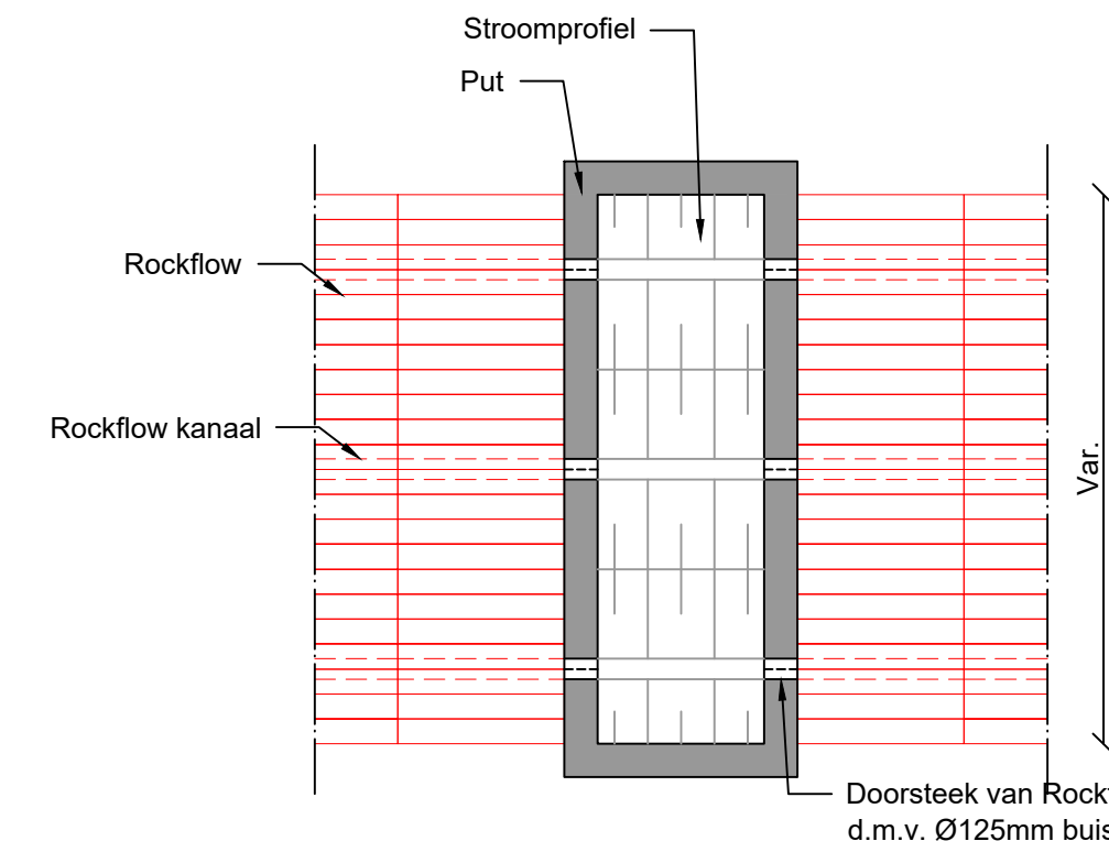
Detail O: Aansluiting Rockflow op put Bovenaanzicht Schaal: 1:50
