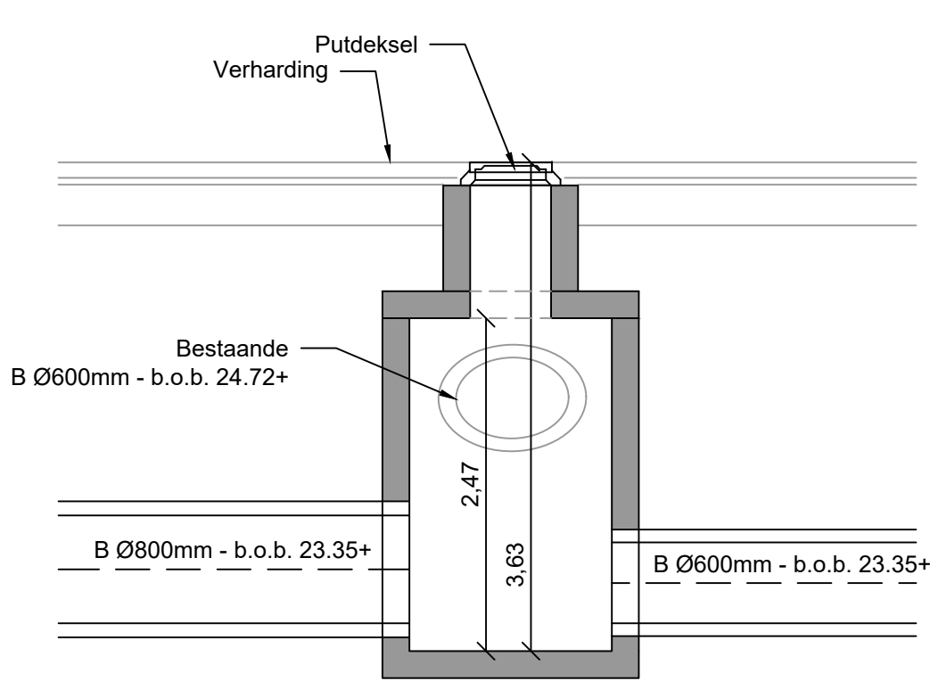
Detail L: Put 05572 Zijaanzicht Schaal: 1:50
