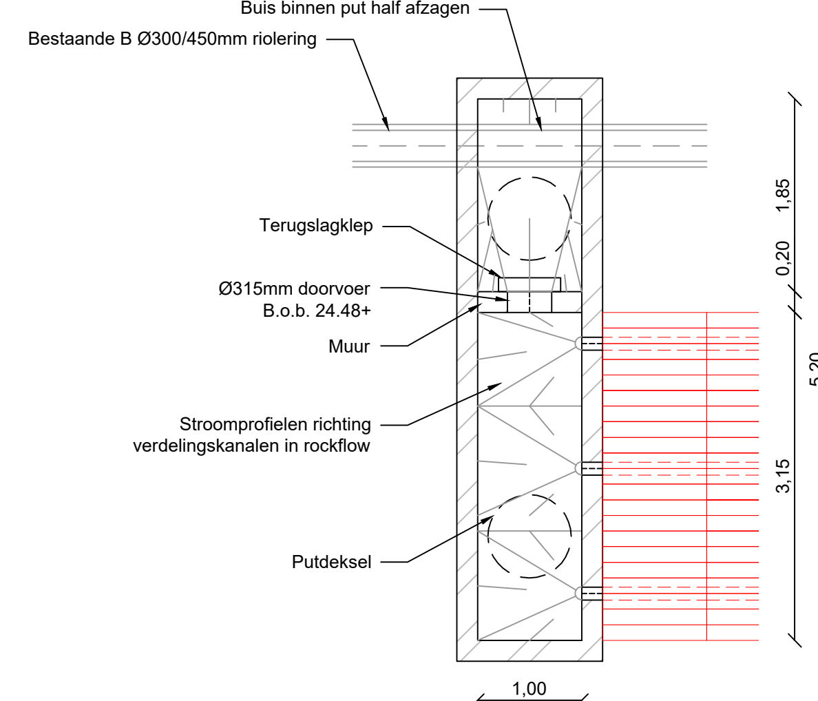
Detail I: Put 05502 Bovenaanzicht Schaal: 1:50
