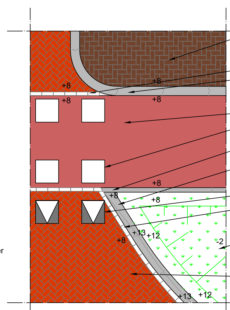
Detail D: Aansluiting elementen op asfalt t.p.v. kruising fietspad Bovenaanzicht Schaal: 1:50
