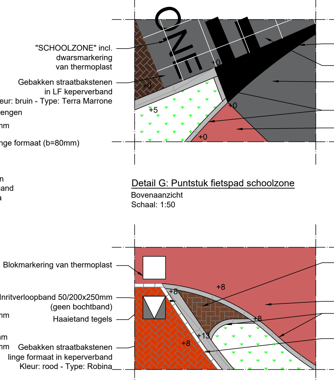
Detail H: Aansluiting kruising fietspad met hoek klinkers Bovenaanzicht Schaal: 1:50
