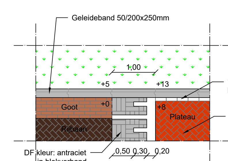
Detail E: Oprit plateau Bovenaanzicht Schaal: 1:50
