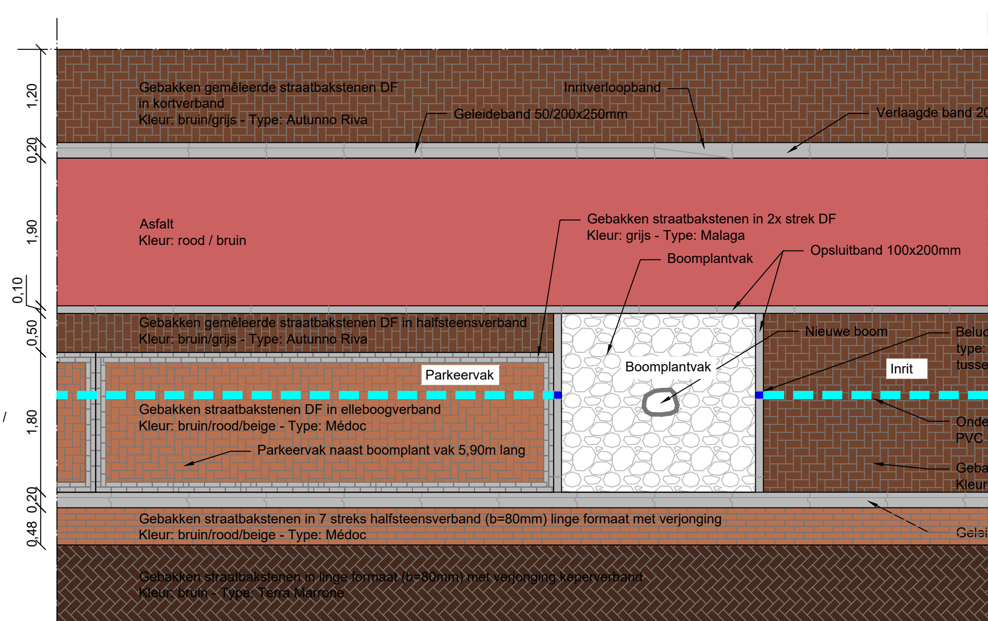
Detail A: Straatwerk Bovenaanzicht Schaal: 1:50
