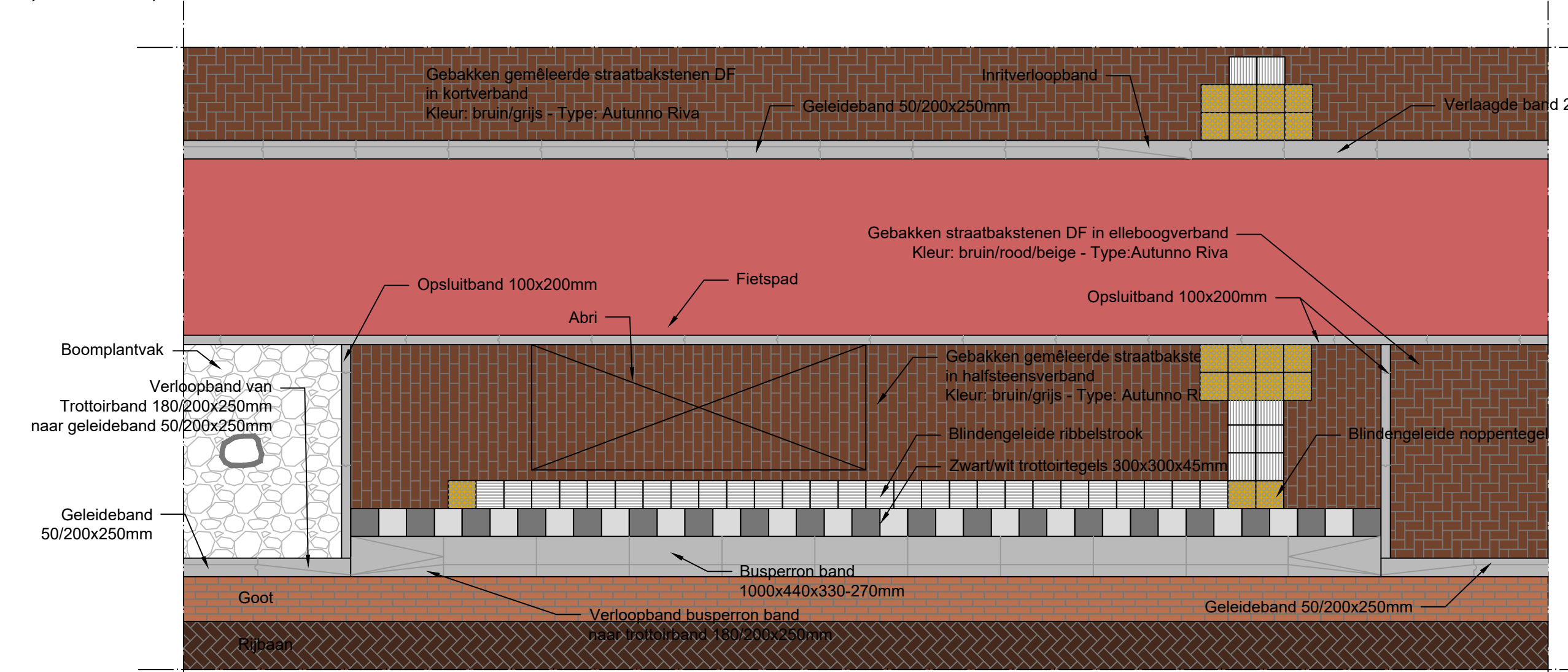
Detail B: Bushalte Bovenaanzicht Schaal: 1:50
