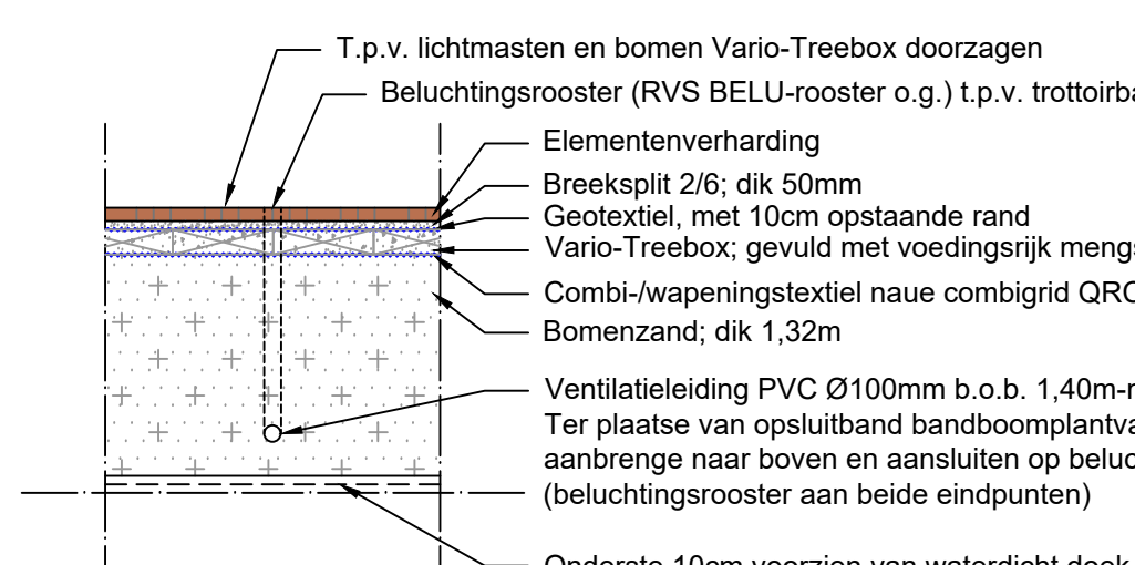
Detail C: Vario-Treebox Zijaanzicht Schaal: 1:50
