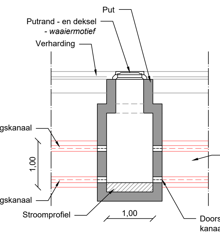
Detail P: Aansluiting Rockflow op put Zijaanzicht Schaal: 1:50
