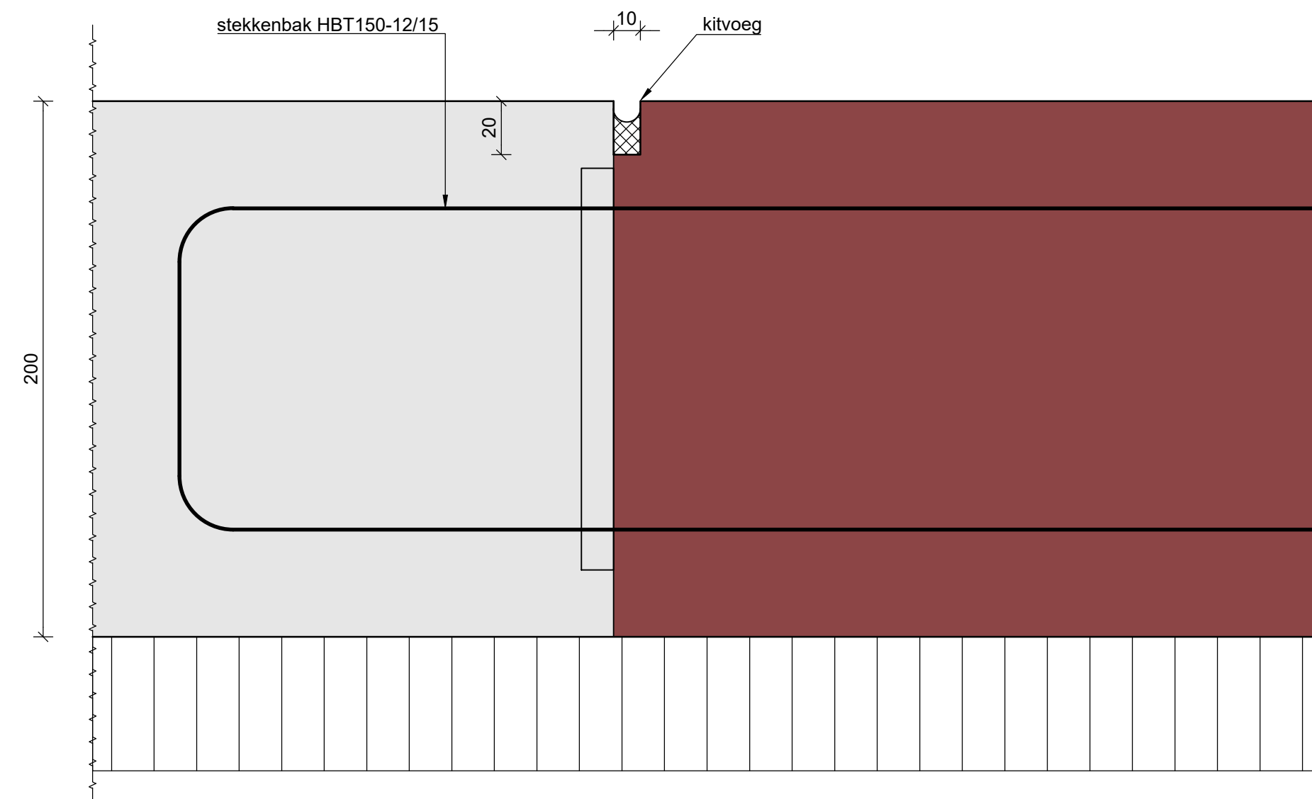
Principedetail sponing schaal: 1:2
