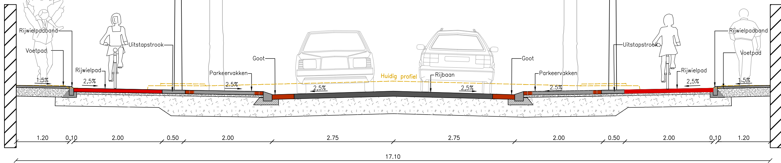
Minimaal profiel Kapellerlaan nieuwe bomen Schaal 1:50
