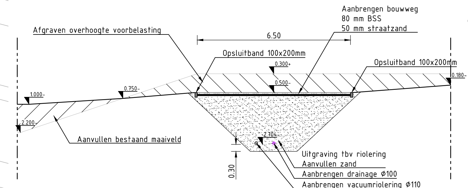
DP-01: Principe profiel bouwweg SCHAAL 1:100
