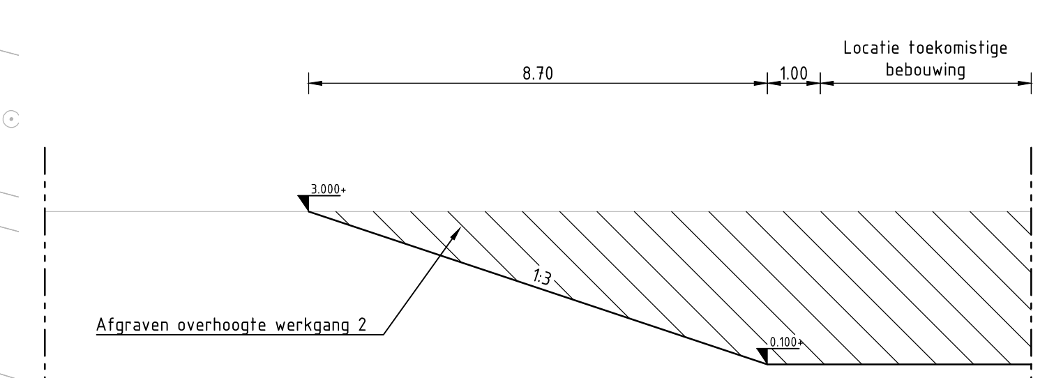
DP-02: Principe profiel afwerkhoogte f.b.v. werkgang 2 SCHAAL 1:100
