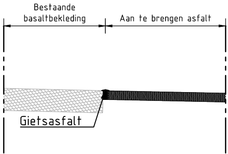
Detail 02: Overgang asfaltverharding met basaltbekleding schaal: 1:50
