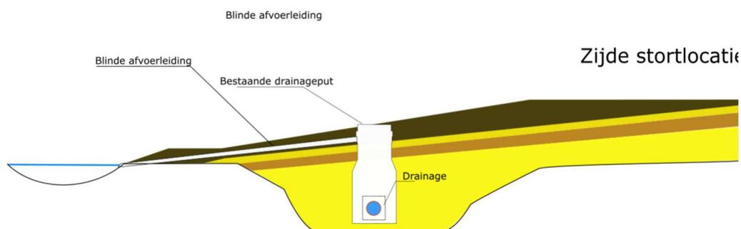
Figuur 1: Ontlasting door afvoer per doorspuitput (lichtbruine laag is zandbentonietlaag)
