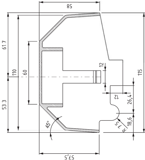
Doorsnede A-A
