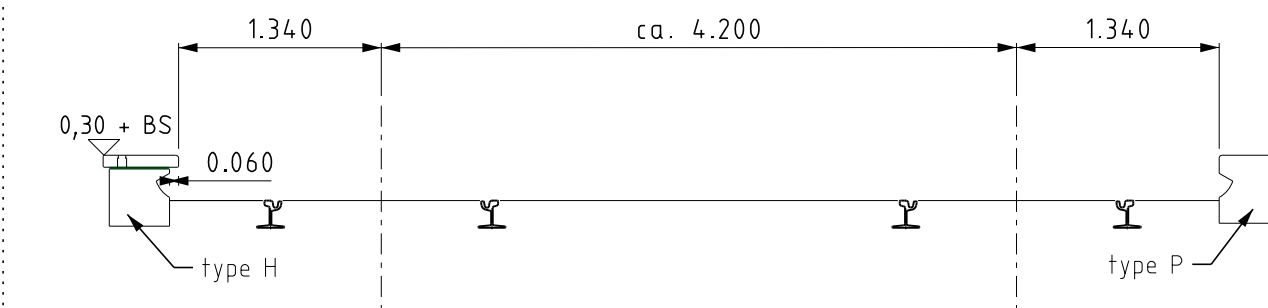
PRINCIPE DOORSNEDE perronband type P en H schaal 1:50
