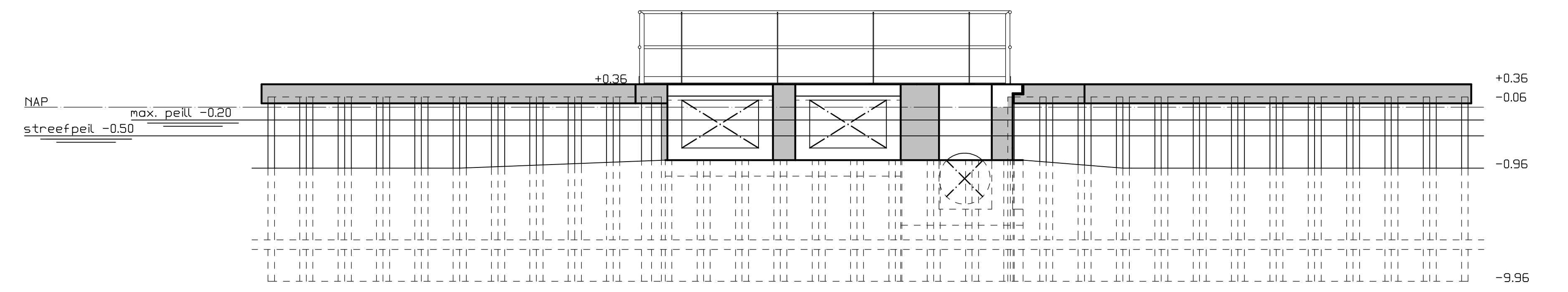
Aanzicht uitstroom 1:50
