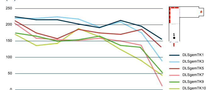
Figuur 7 Temperatuurverloop blussing DLS, gemiddelde waarden per thermokoppel (TK)
