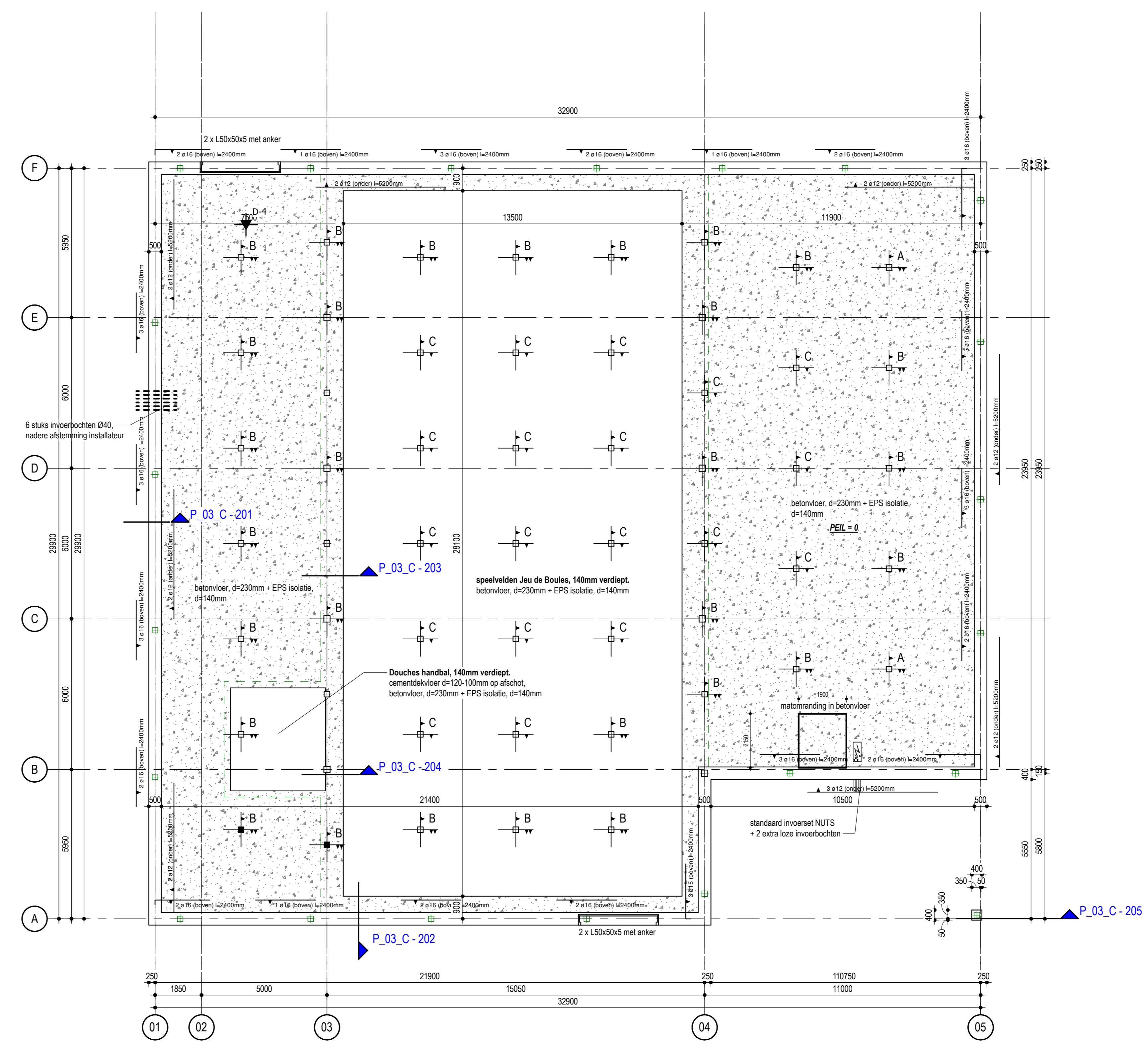
Fundering Begane grondvloer constructief 1:10
