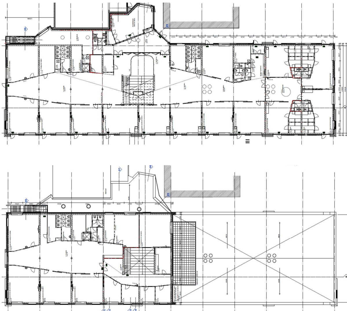
Afbeelding 4 & 5: Plattegronden
