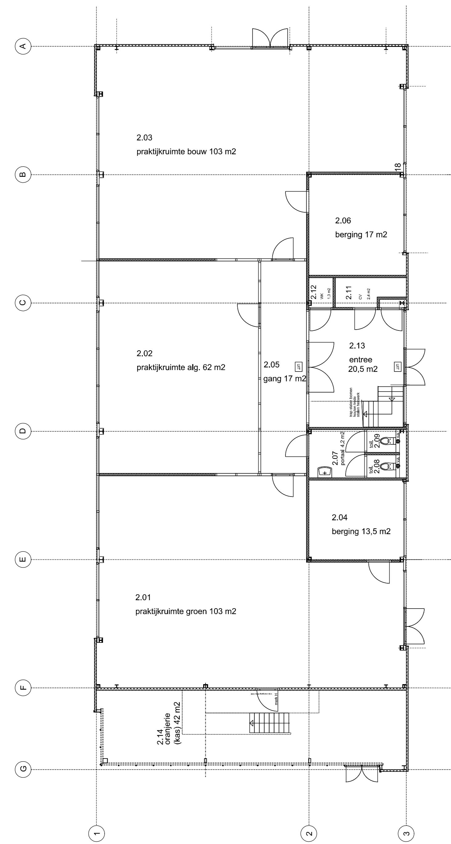
NIEUWBOUW PLATTEGROND BEGANE GROND
