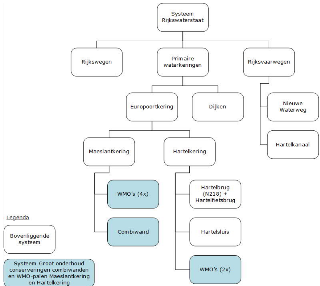
Figuur 4: Systeem 'Groot onderhoud conserveringen combiwanden en WMO-palen Maeslantkering en WMO-Hartelkering' als onderdeel van het grotere systeem
