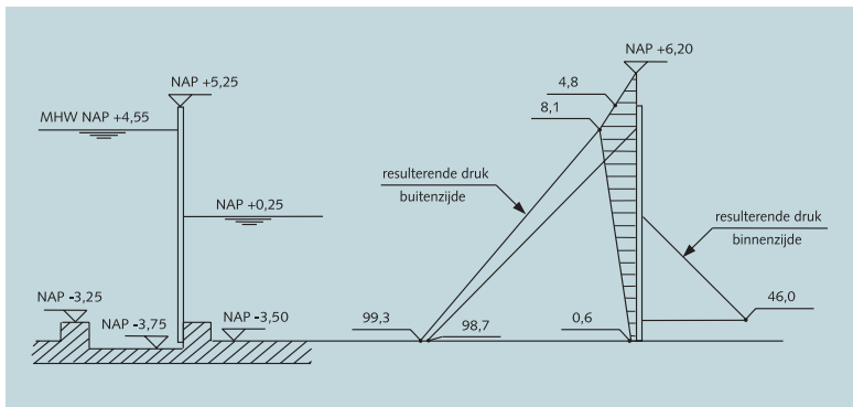
Figuur B9.2 Golfdrukken op deuren buitenhoofd
