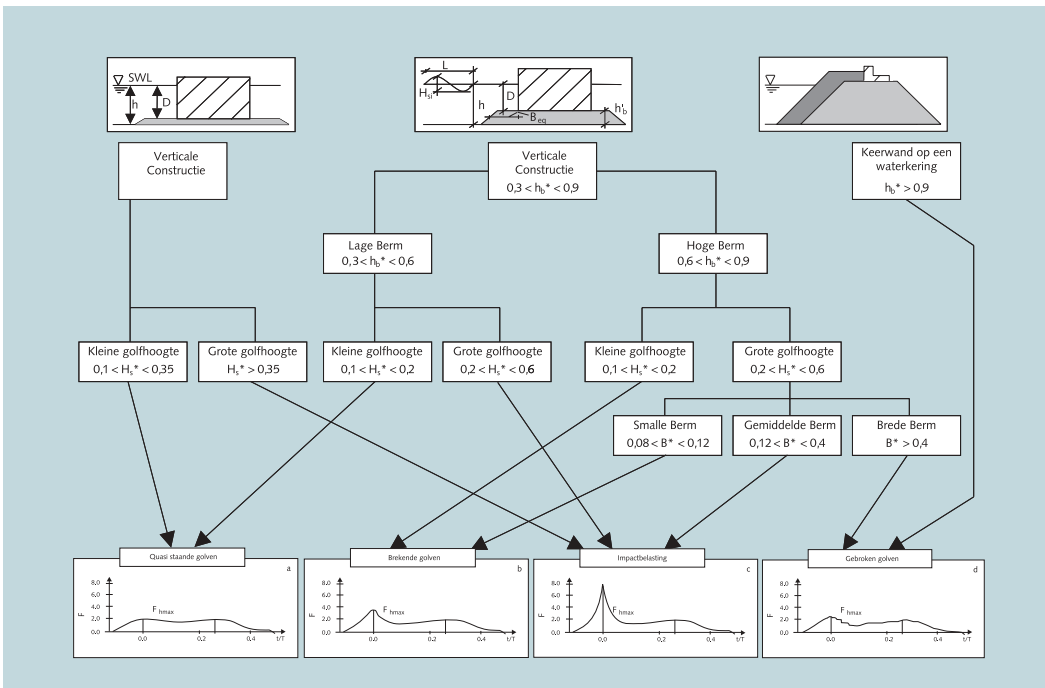
Figuur B5.5 Classificatie golfbelasting, volgens [ref. B5.6]
