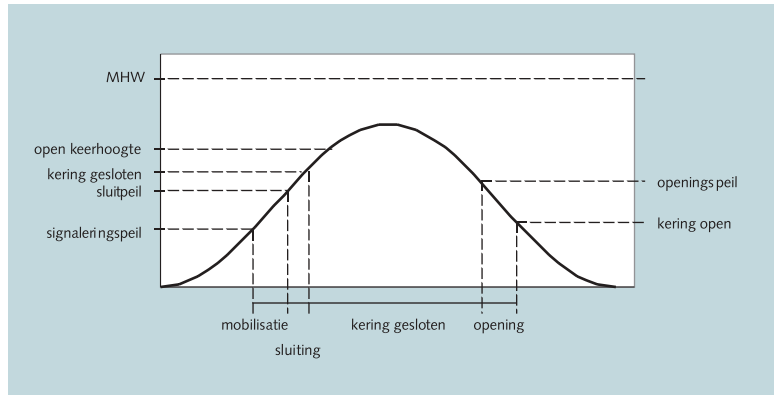
Figuur B3.3 Waterstandsverlooptlijn en belangrijkste peilen
