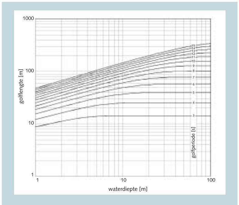
Figuur B5.4 Golflengte als functie van de waterdiepte en de golfterie
