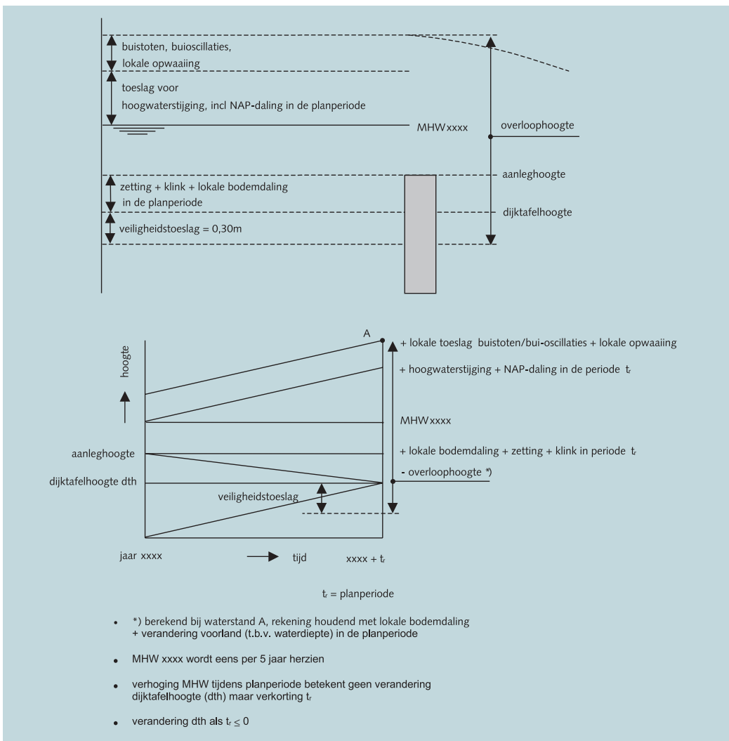
Figuur B2.3 Bijdragen aan de aanleghoogte bij overlopen
