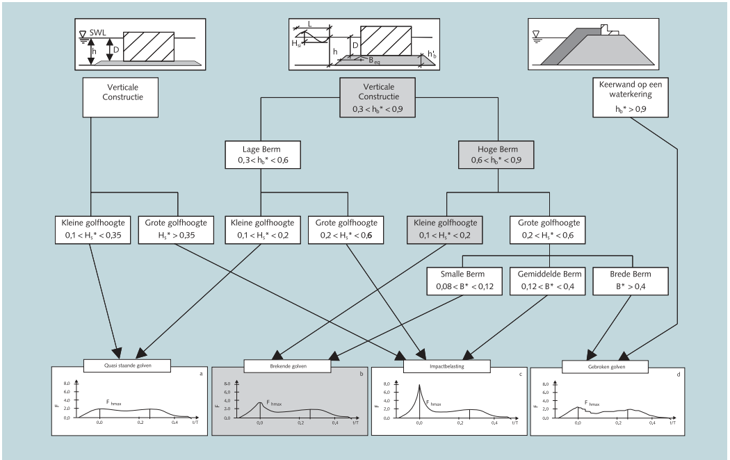
Figuur B5.9 Keuze belastingmodel voorbeeld coupure
