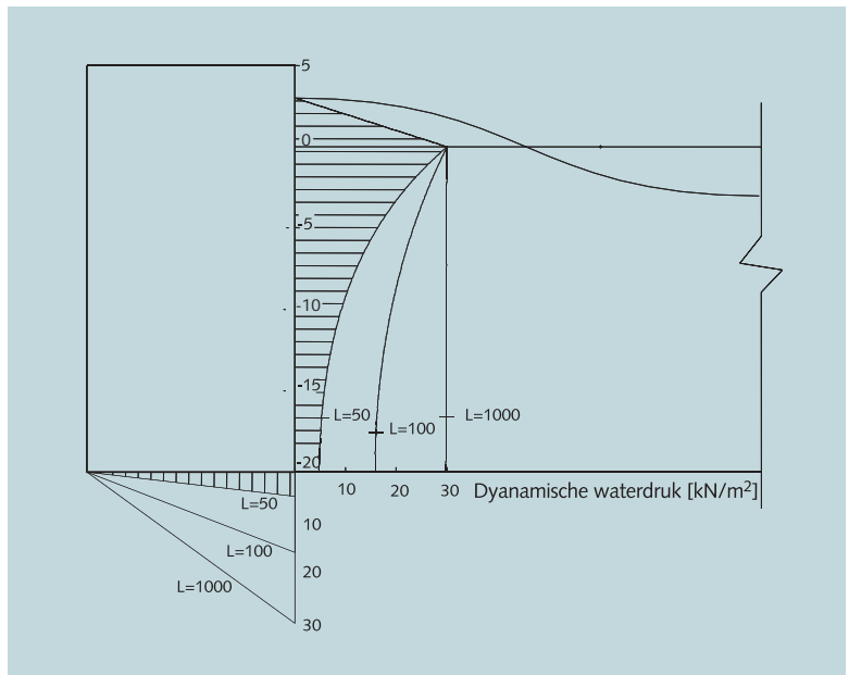
Figuur B5.1 Golfdruk volgens de lineaire golftheorie
