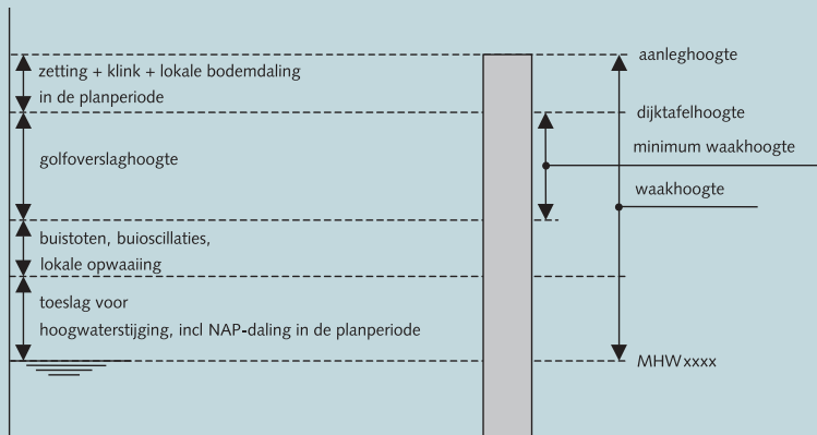
Figuur B2.2 Bijdragen aan de aanleghoogte bij golfoverslag
