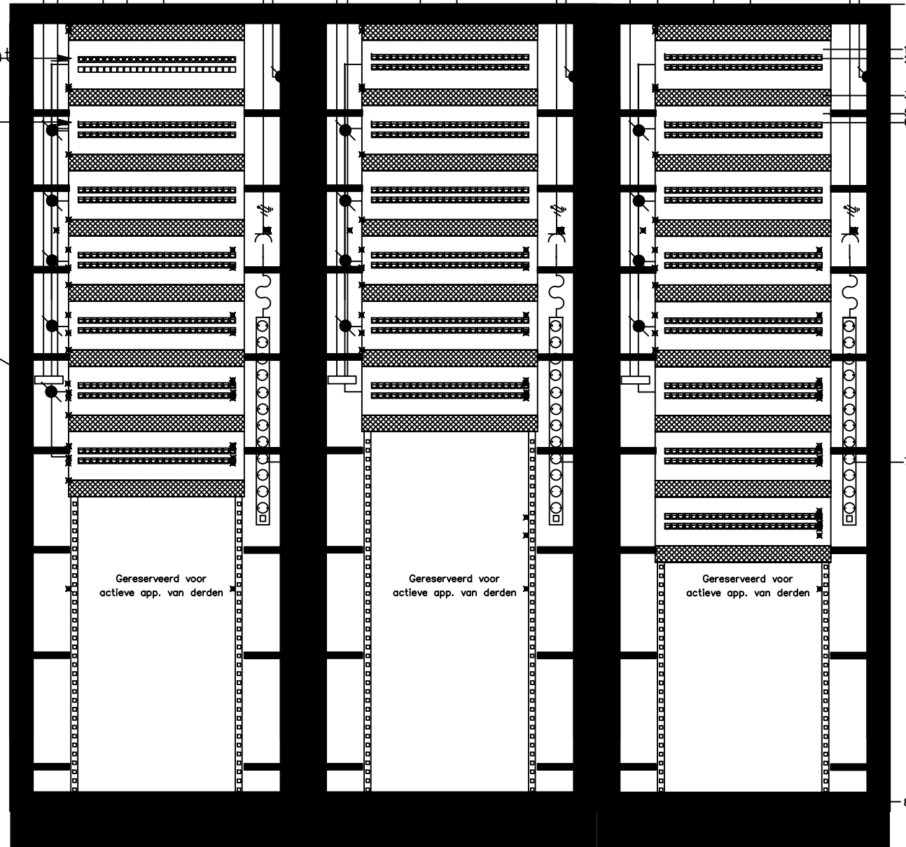
distributiepaneel DP0.1 werkplekken verdieping distributiepaneel DP0.2 telefoon distributiepaneel DP0.3 werkplekken begane grond
