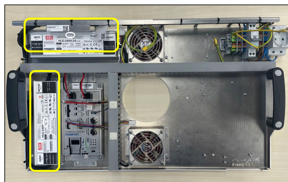
Figuur 4-6: Slave-variant, voedingen gemarkeerd.
