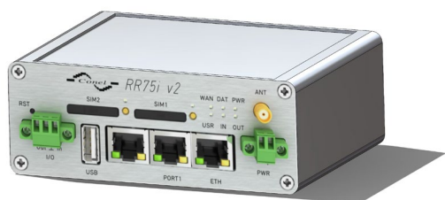
Figuur 4-13: GSM-R-modem (vooraanzicht)
