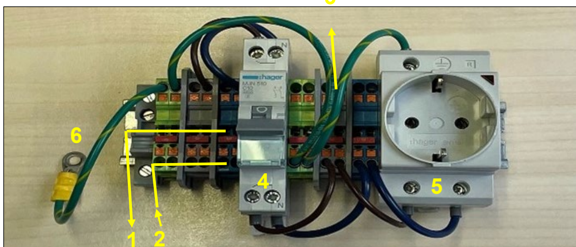
Figuur: 4-28: DIN-assemblage
