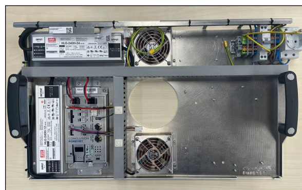
Figuur 4-16: Slave-variant.
