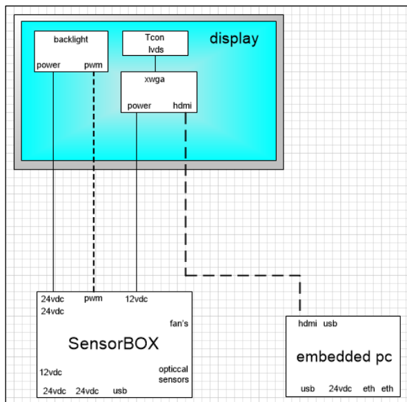
Figuur 4-30: Paneel aansluitschema
