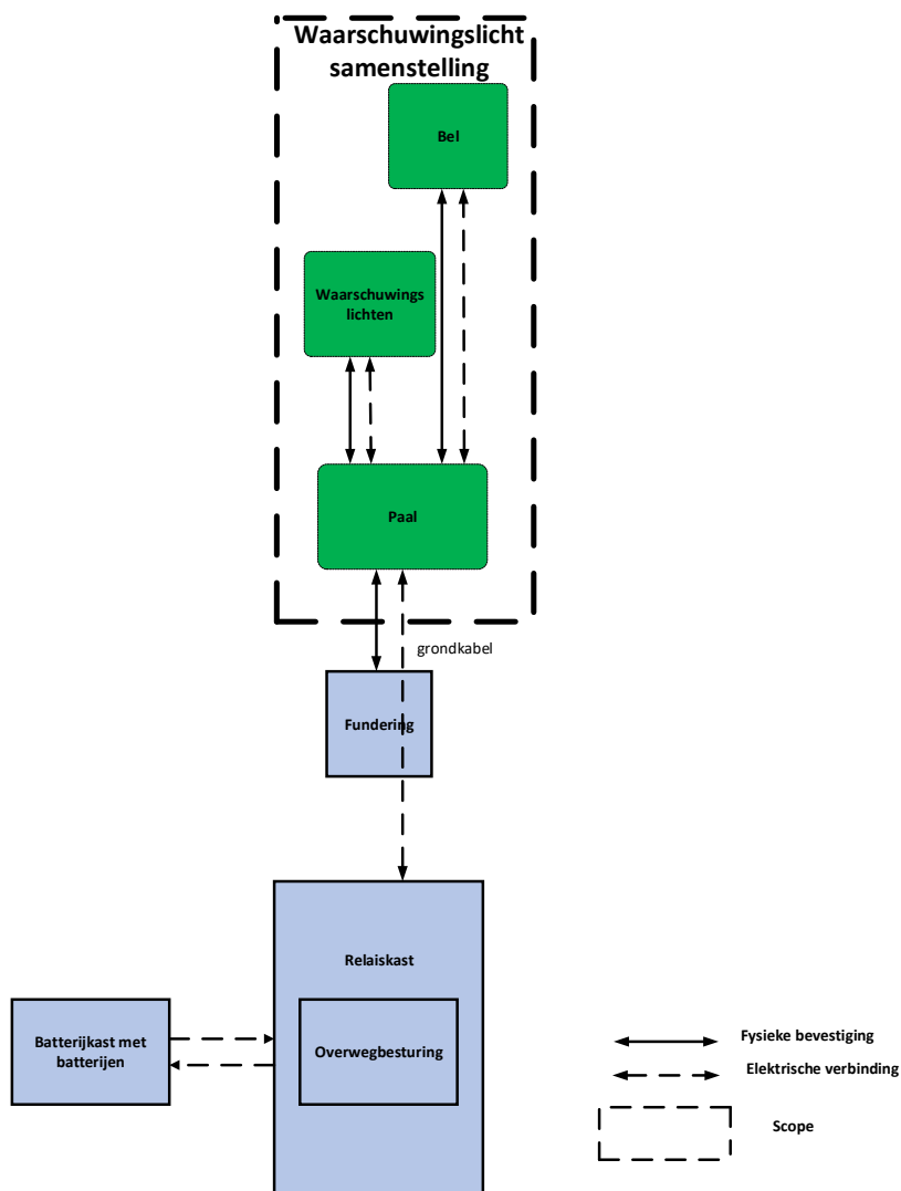
Figuur 1: Systeemgrenzen waarschuwing licht samenstelling
