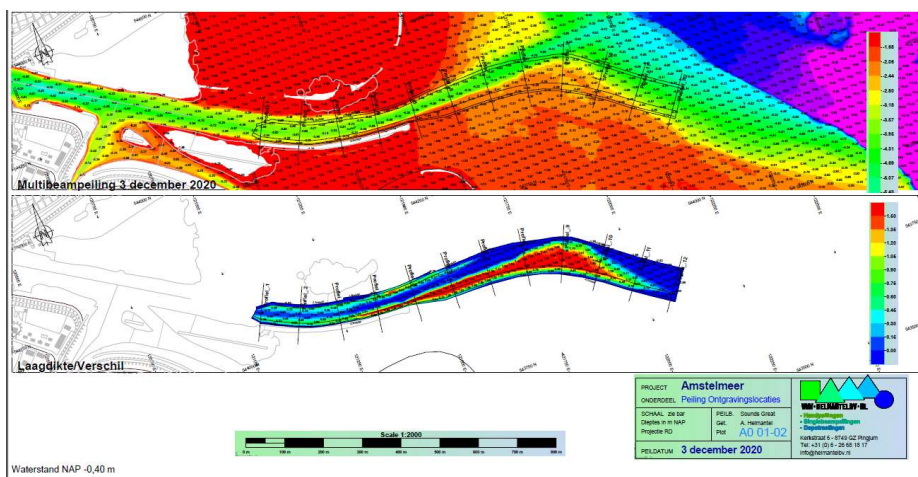
Abbeelding 2.5b: Verdeling van de aanzanding over de baggervakken locatie 2 (Balgzand) (op basis van: multibeam peiling – leggerprofiel)
