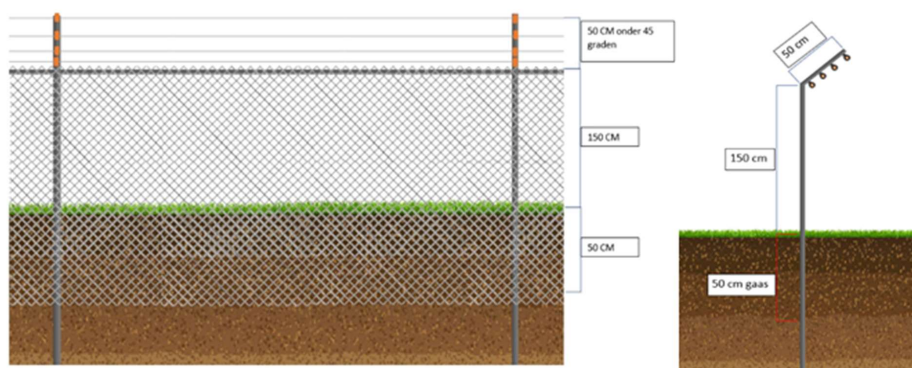
Tekening 5a: Dwarsdoorsnede en aanzicht hekwerk
