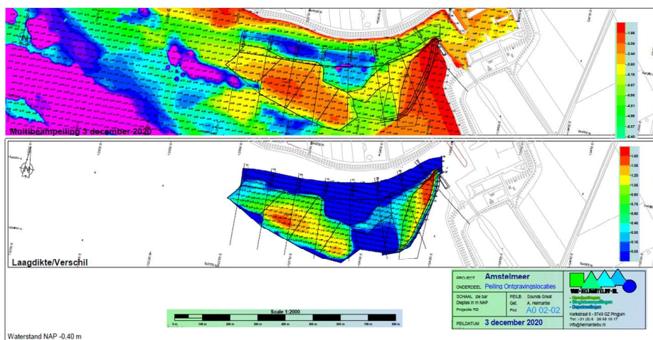
Abbeelding 2.5a: Verdeling van de aanzanding over de baggervakken locatie 1 (De Haukes) (op basis van: multibeam peiling – leggerprofiel)
