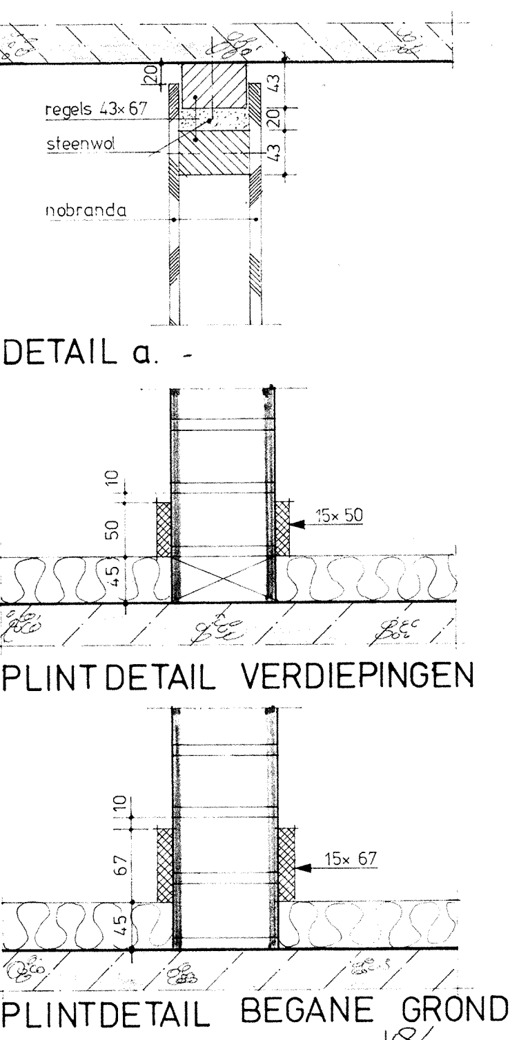
PLINTDETAIL BEGANE GROND
