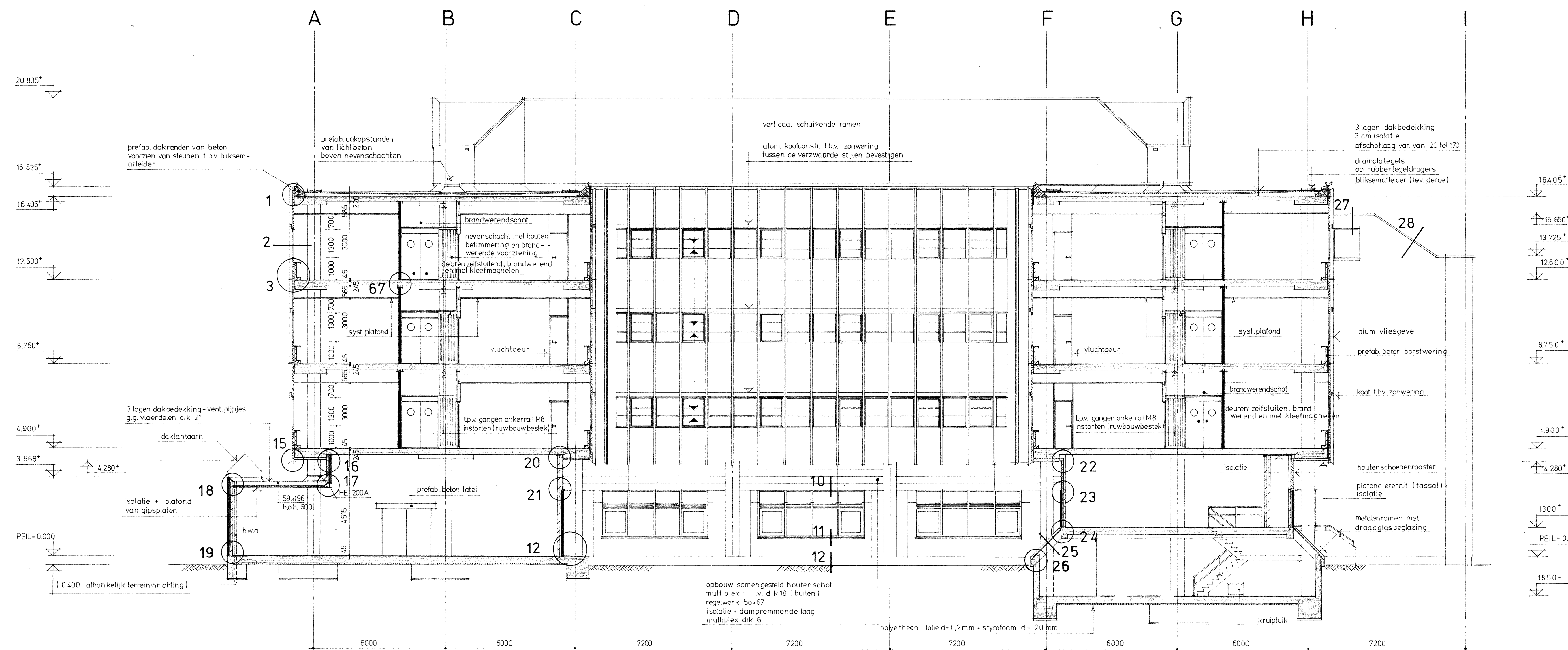
DOORSNEDE B - B.
