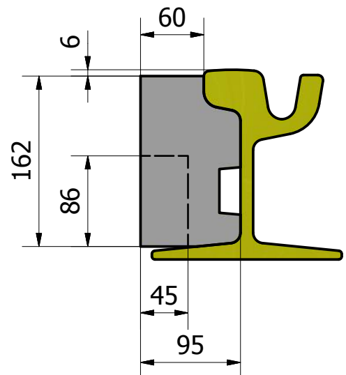
Querschnitt ( 1 : 5 )
