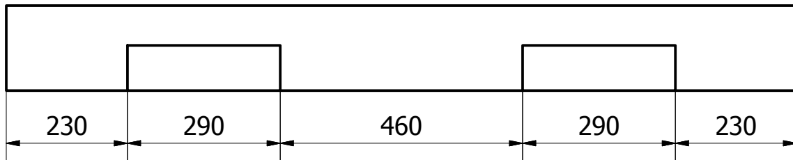
Vorderansicht ( 1 : 10 )
