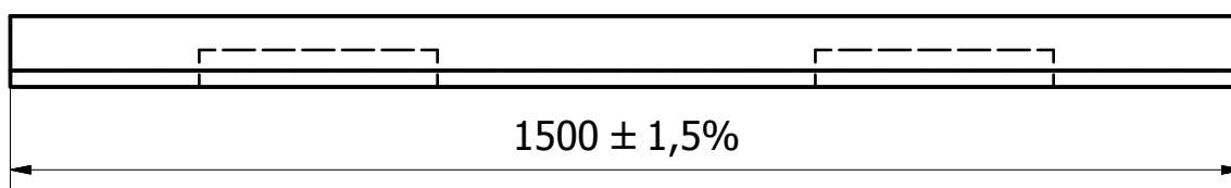
Querschnitt ( 1 : 5 )
