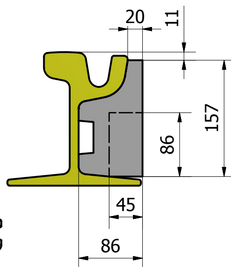
Querschnitt ( 1 : 5 )
