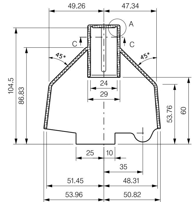
Doorsnede B-B
