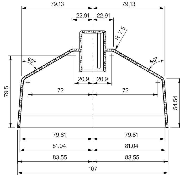
Doorsnede A-A
