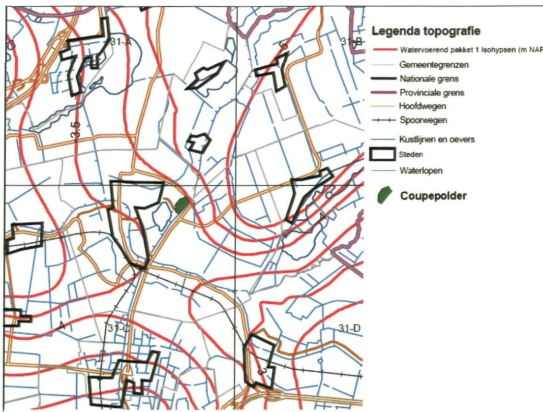
Figuur 2: Uitsnede uit berekend isohypsenspatroon eerste watervoerend pakket omgeving Alphen a/d Rijn, situatie april 1995 (TNO, 2002).
