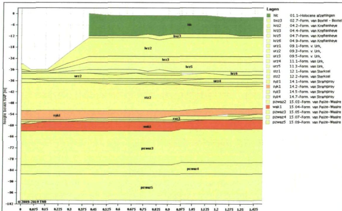
Figuur 2.2 ZW-NO hydrogeologisch profiel vanuit Zegerplas over Coupépolder (TNO, 2010)
