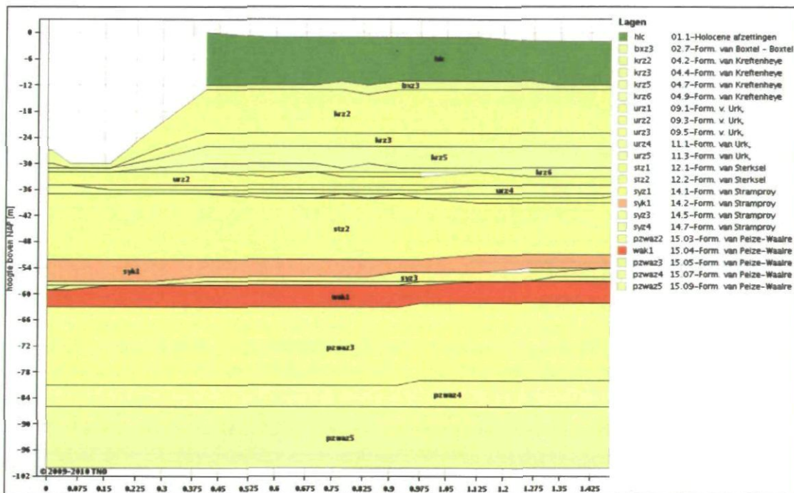
Figuur 1: ZW-NO hydrogeologisch profiel vanuit Zegerplas over Coupépolder (TNO, 2010).
