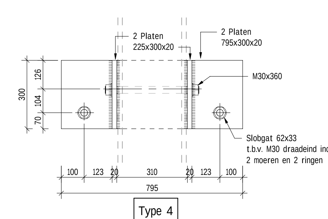
AANZICHT CONSOLES TYPE 4 schaal: 1 : 10
