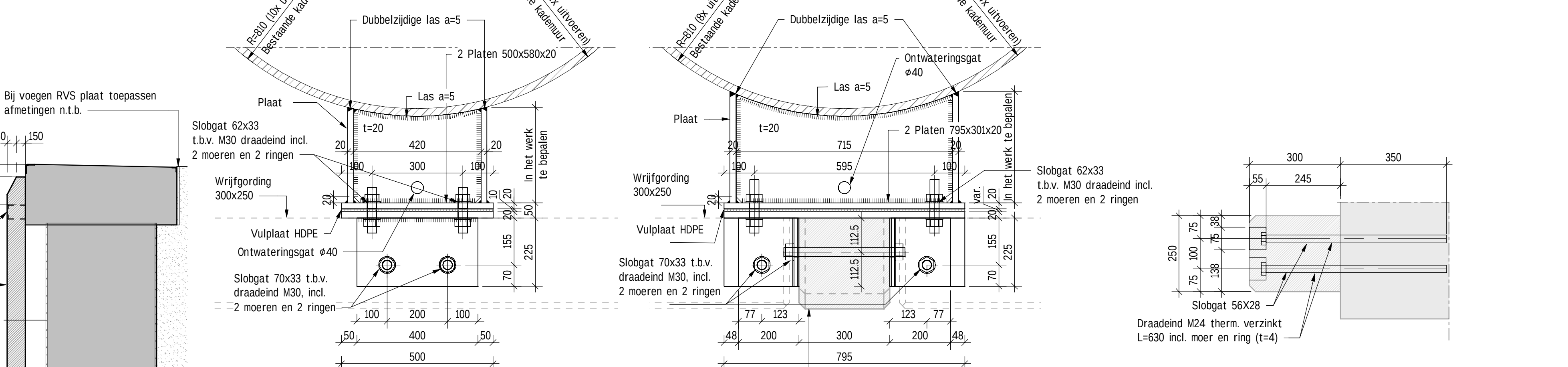
BEVESTIGING AAN DEKSLOOF schaal: 1 : 10
