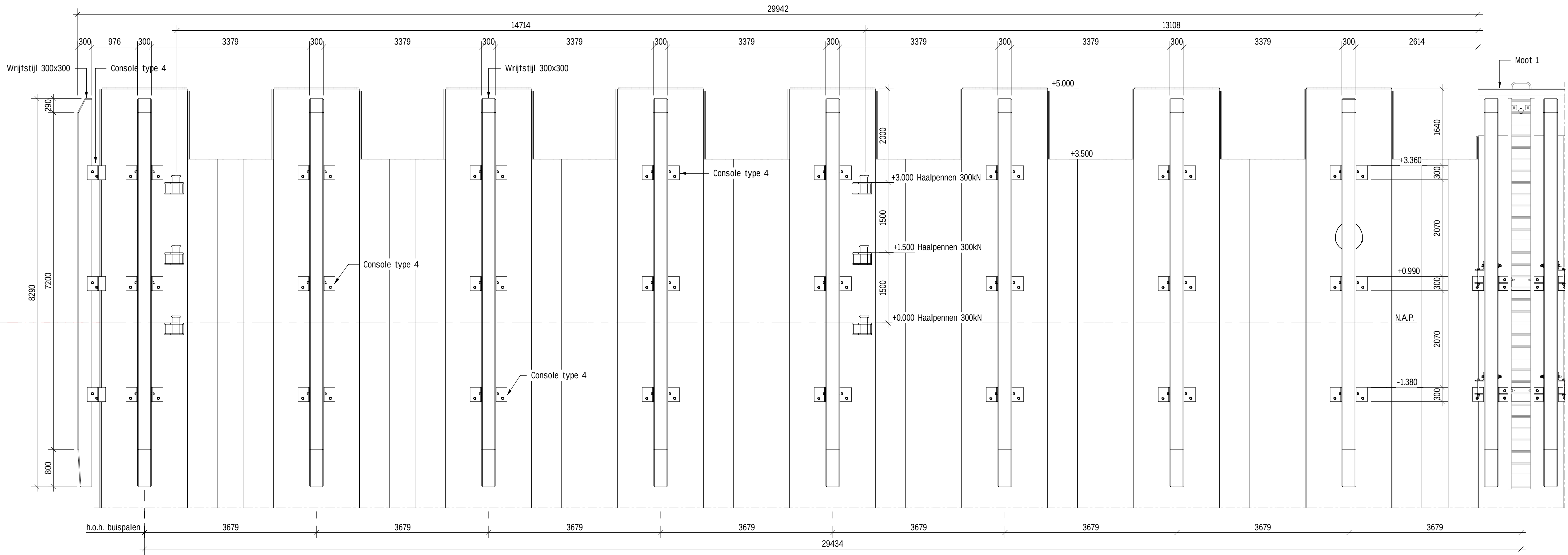
VOORAANZICHT VLEUGELWAND schaal: 1 : 50
