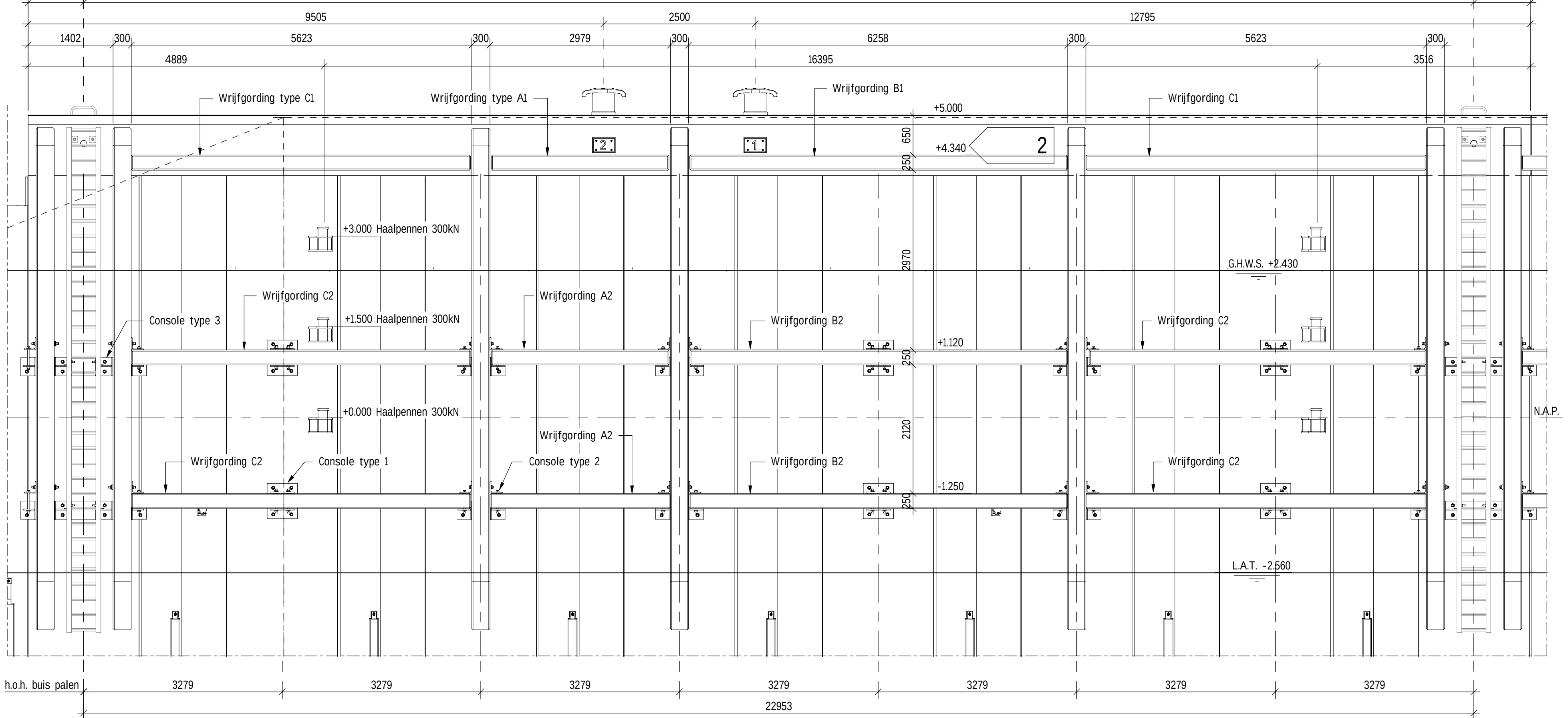
VOORAANZICHT MOOT 1 schaal: 1 : 50
