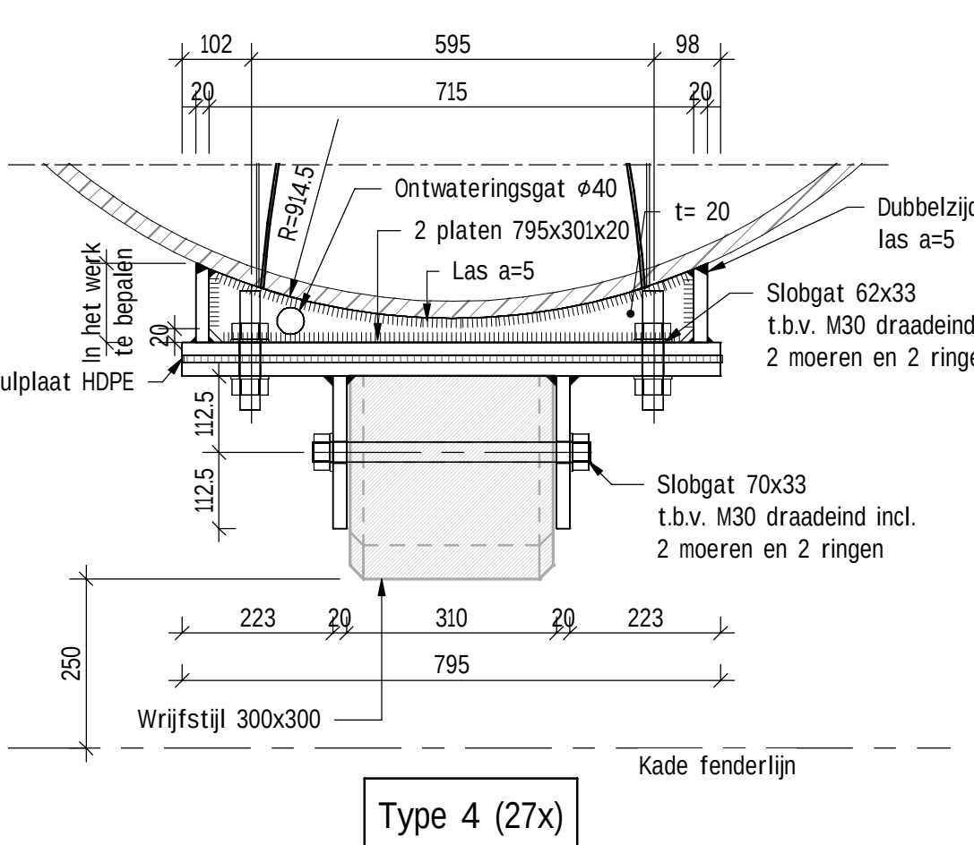
PRINCIPE DETAIL CONSOLES - VLEUGELWAND schaal: 1 : 10
