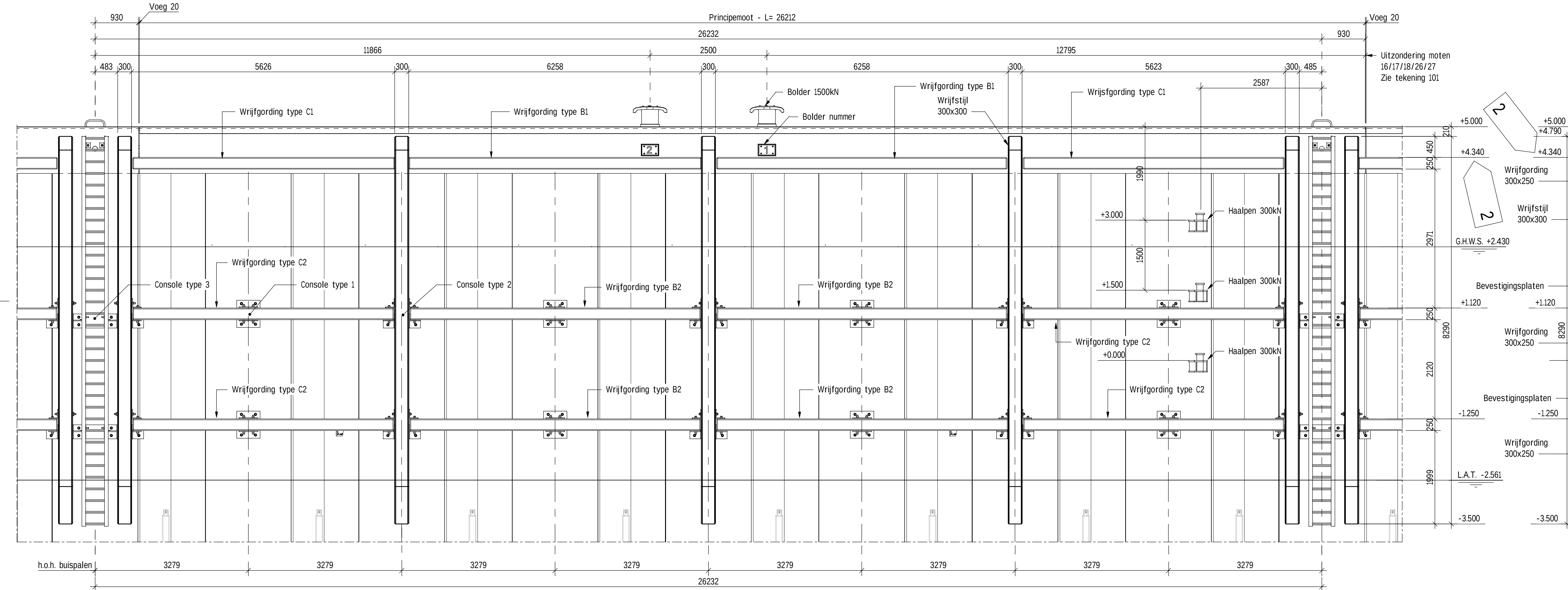
PRINCIPEMOOT schaal: 1 : 50
