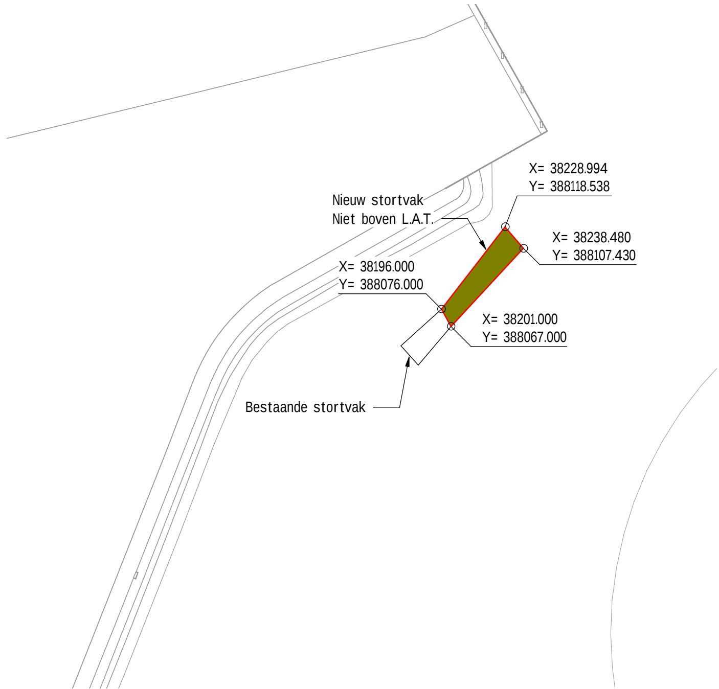
GEBIED A schaal: 1 : 2000
