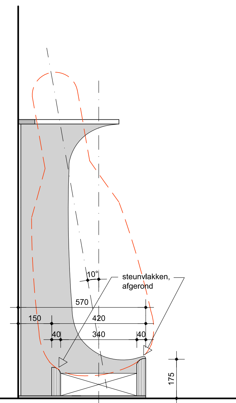
doorsnede
