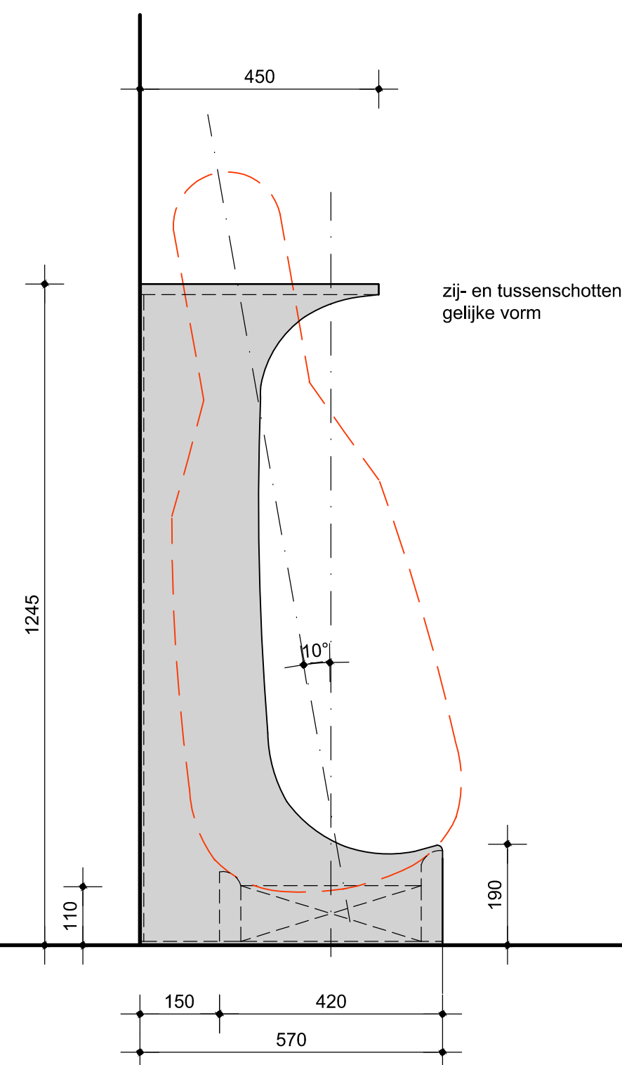
zijaanzicht
