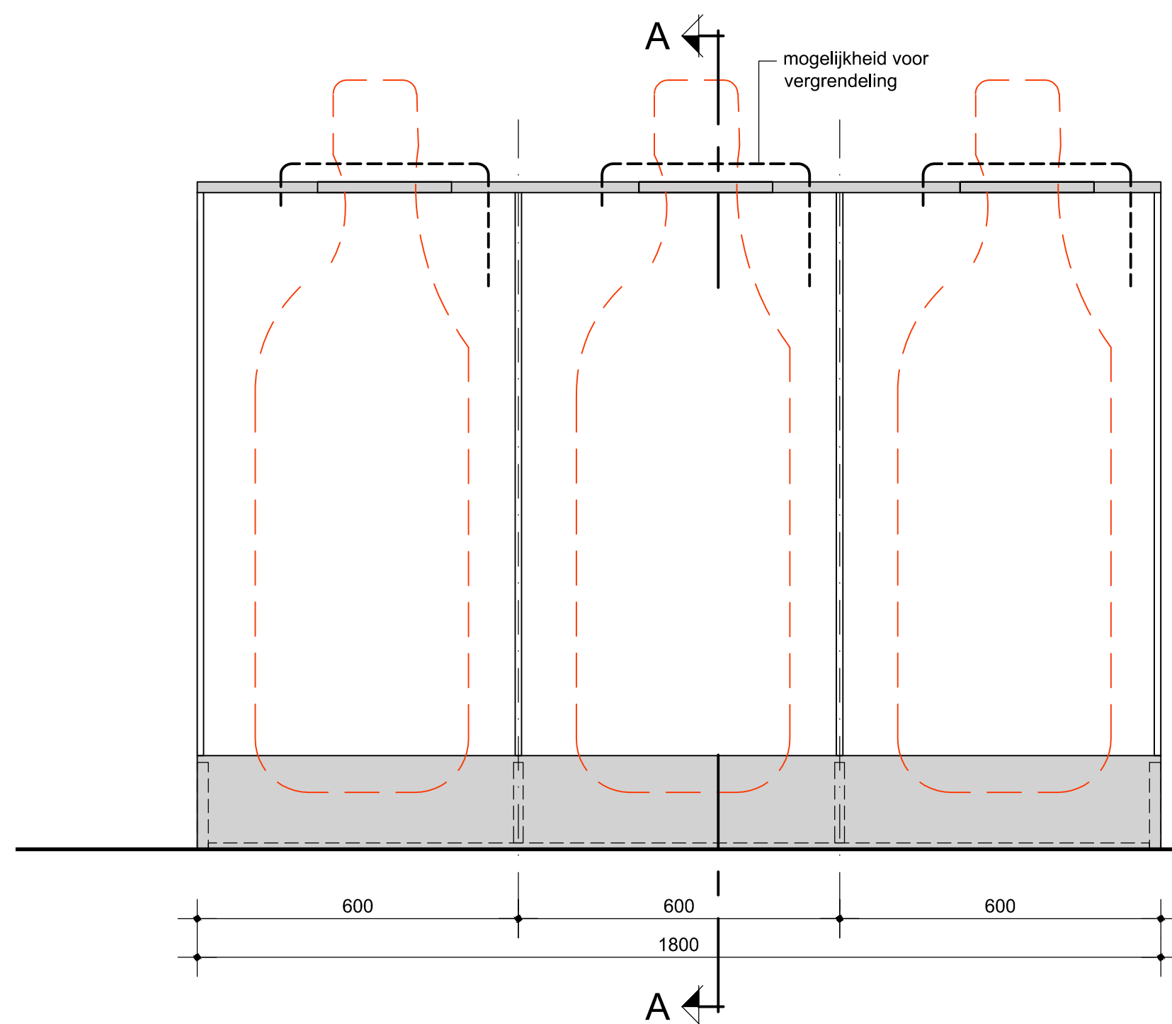
vooraanzicht
