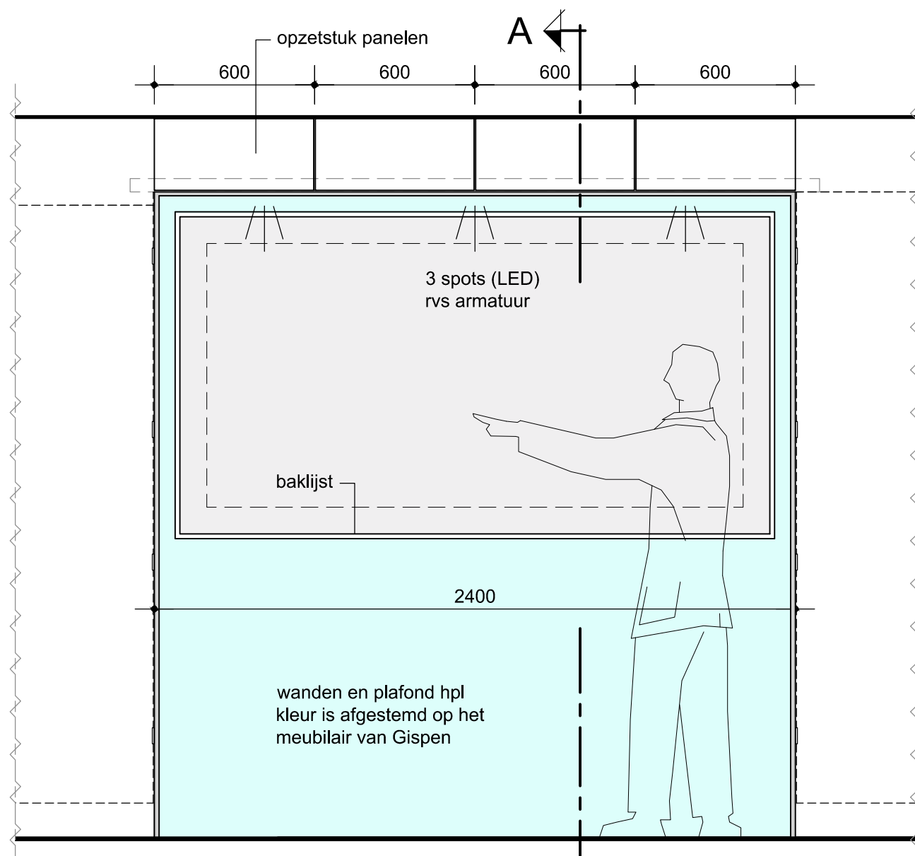
vooraanzicht
