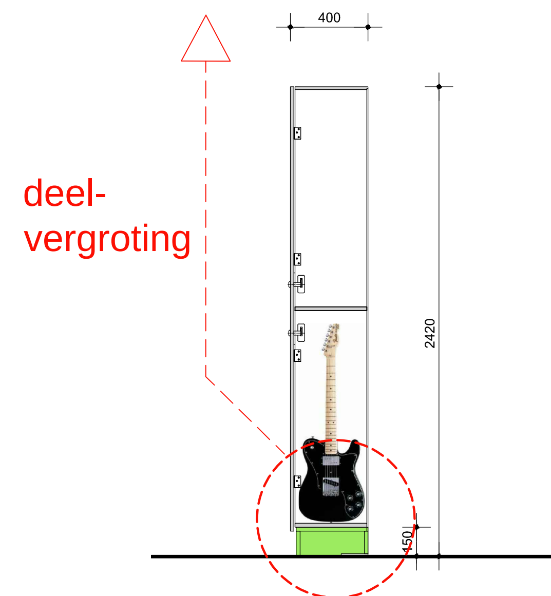
drsn. A-A (1:20)
