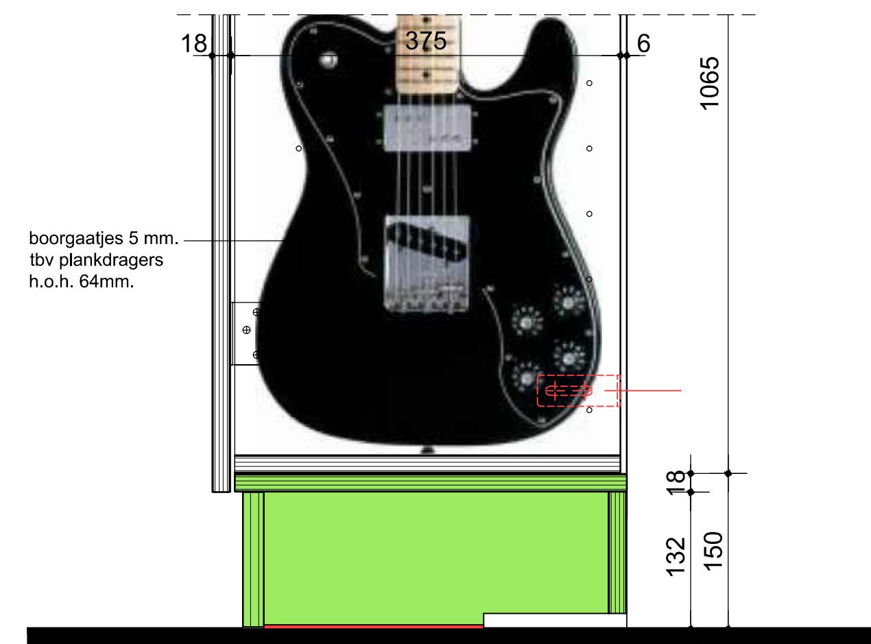
kast (deelvergroting) 1:5
