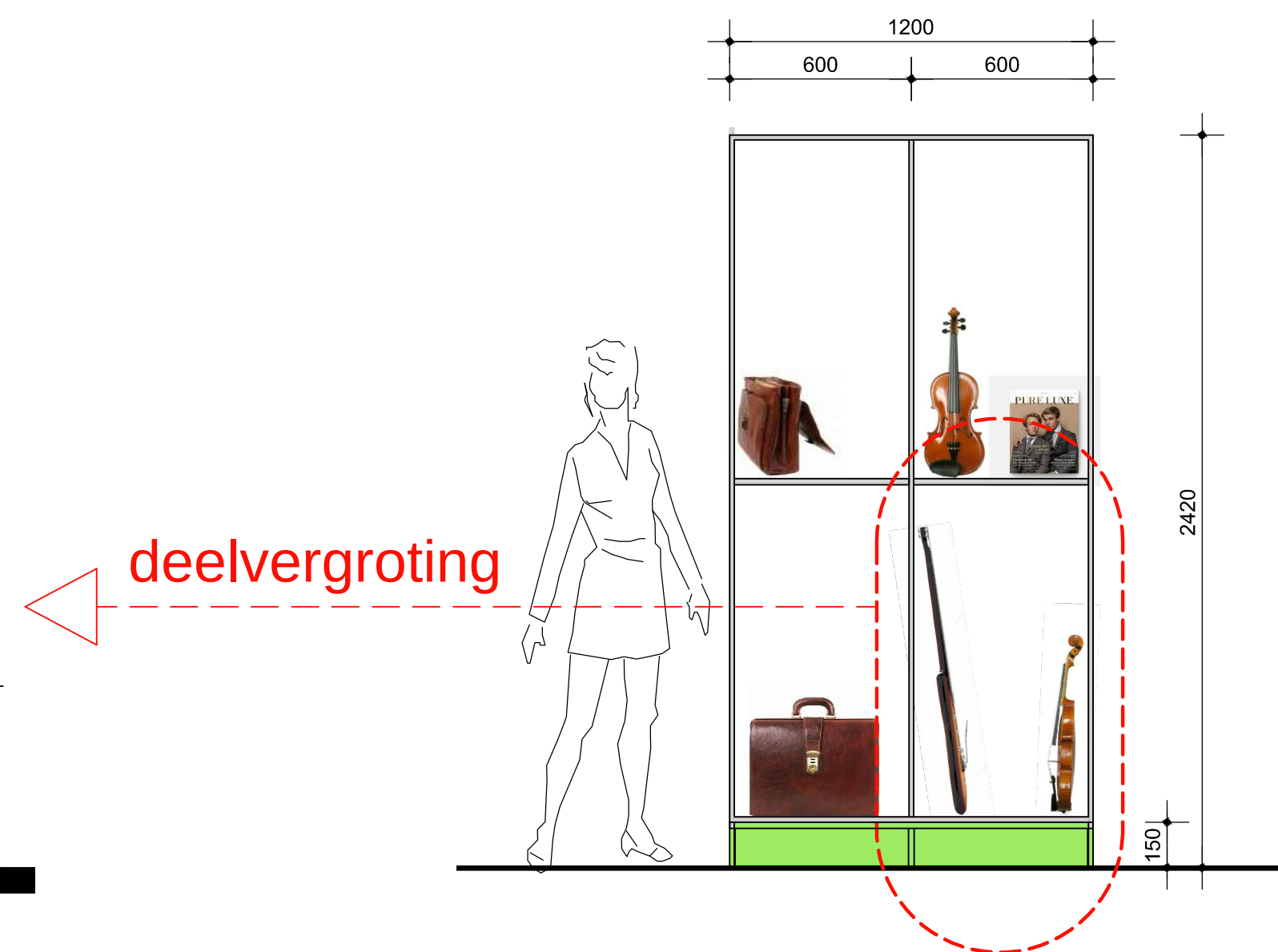
binnenaanzicht (1:20)
