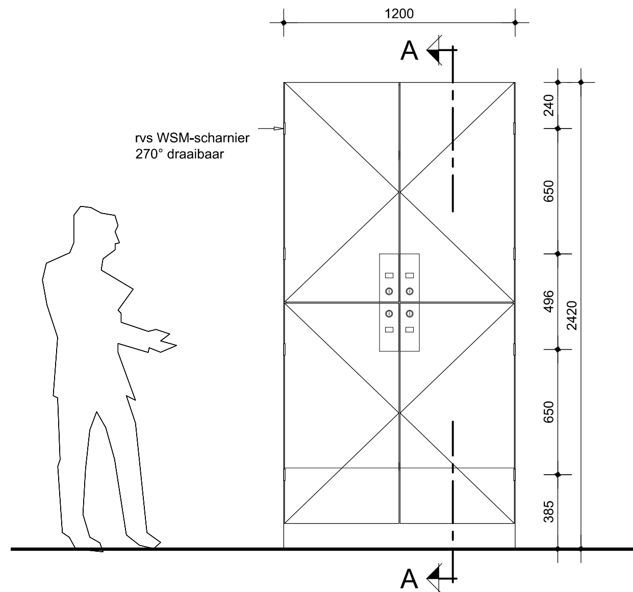
vooraanzicht (1:20)
