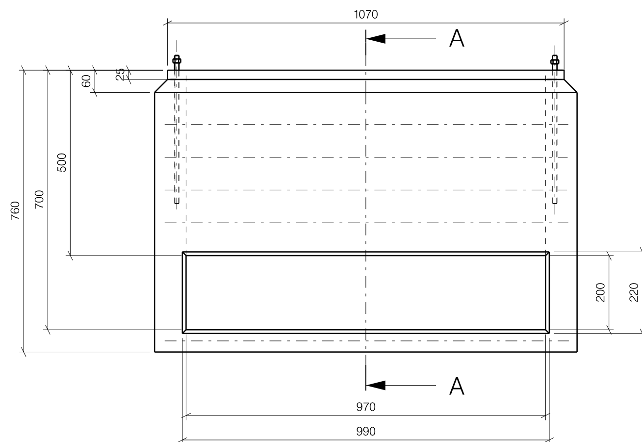
Vooraanzicht
