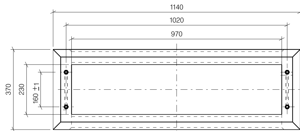
Bovenaanzicht
