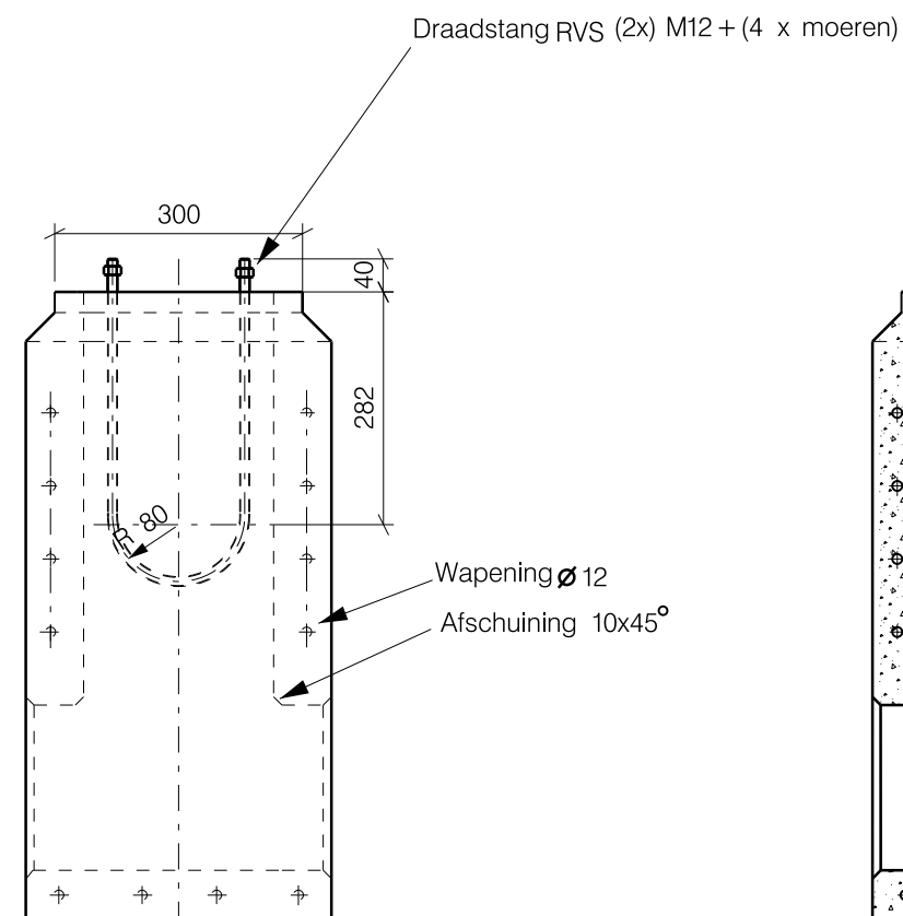
Zijaanzicht
