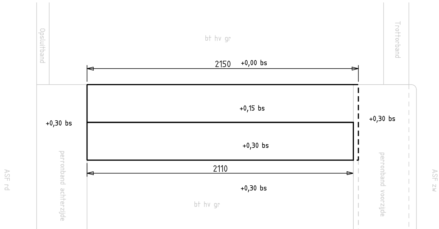
Bovenaanzicht
