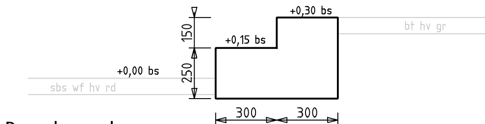
Dwarsdoorsnede
