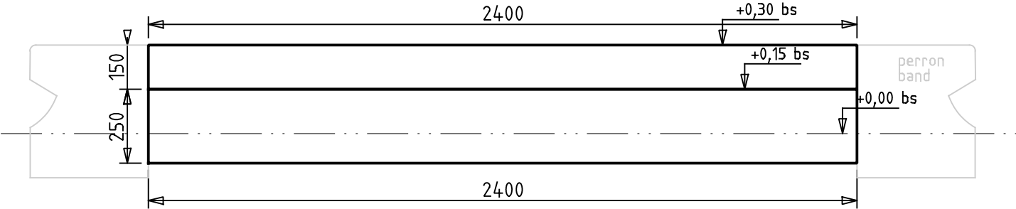
vooraanzicht
