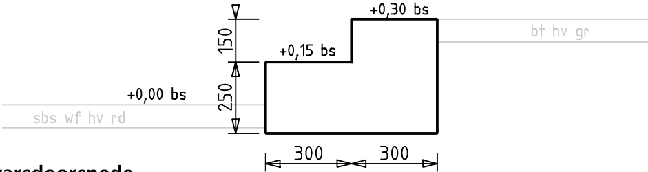
Dwarsdoorsnede
