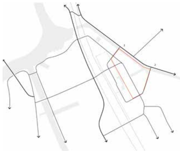
7. voorstel fietsnetwerk
