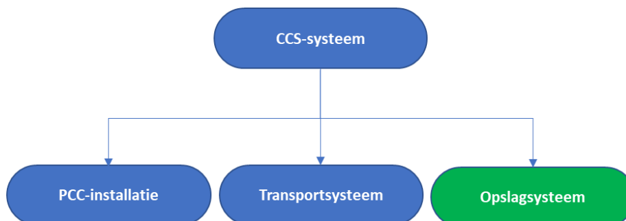
Afbeelding 2.4 Objectenboom CCS-systeem
